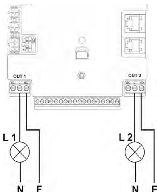
Afbeelding 10: Voorbeeld van aansluiting van de uitgangen
