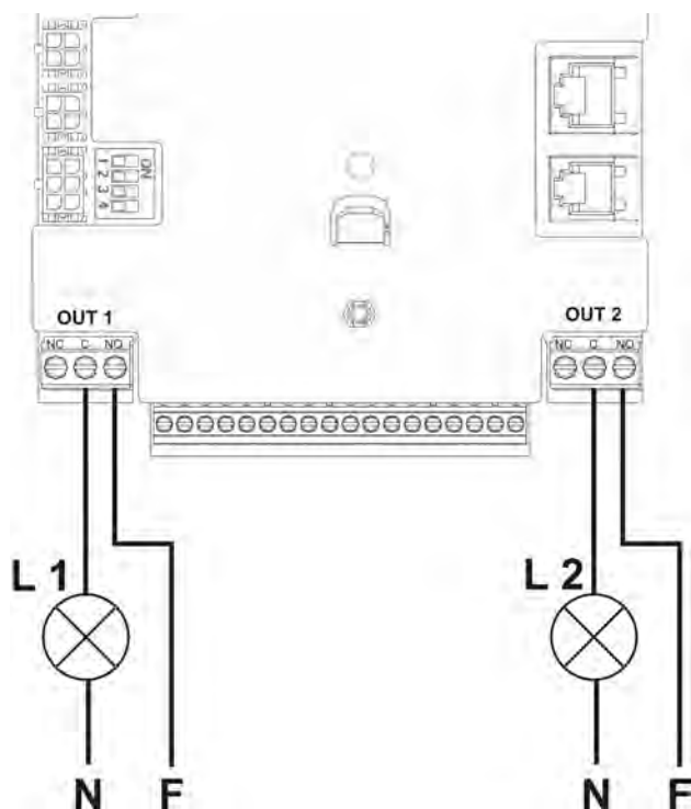
Figure 10: Exemple de connexion des sorties
