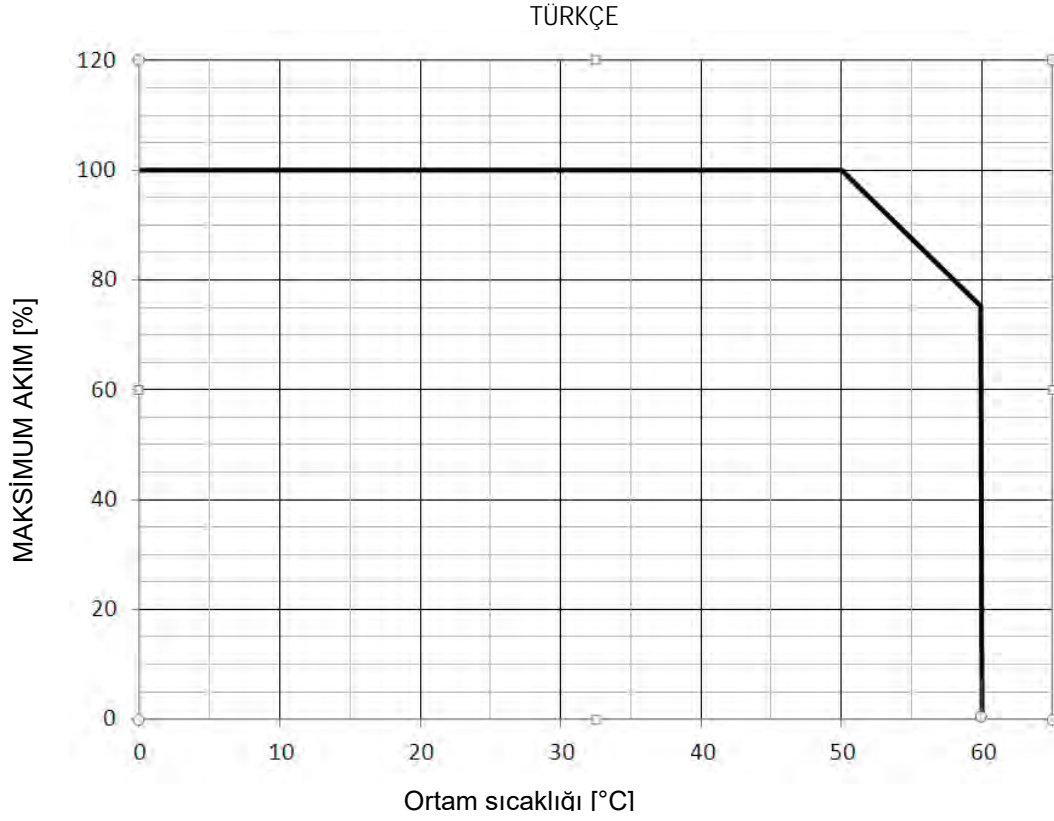
Şekil 1:Ortam sıcaklığına göre akım azalma eğrisi
