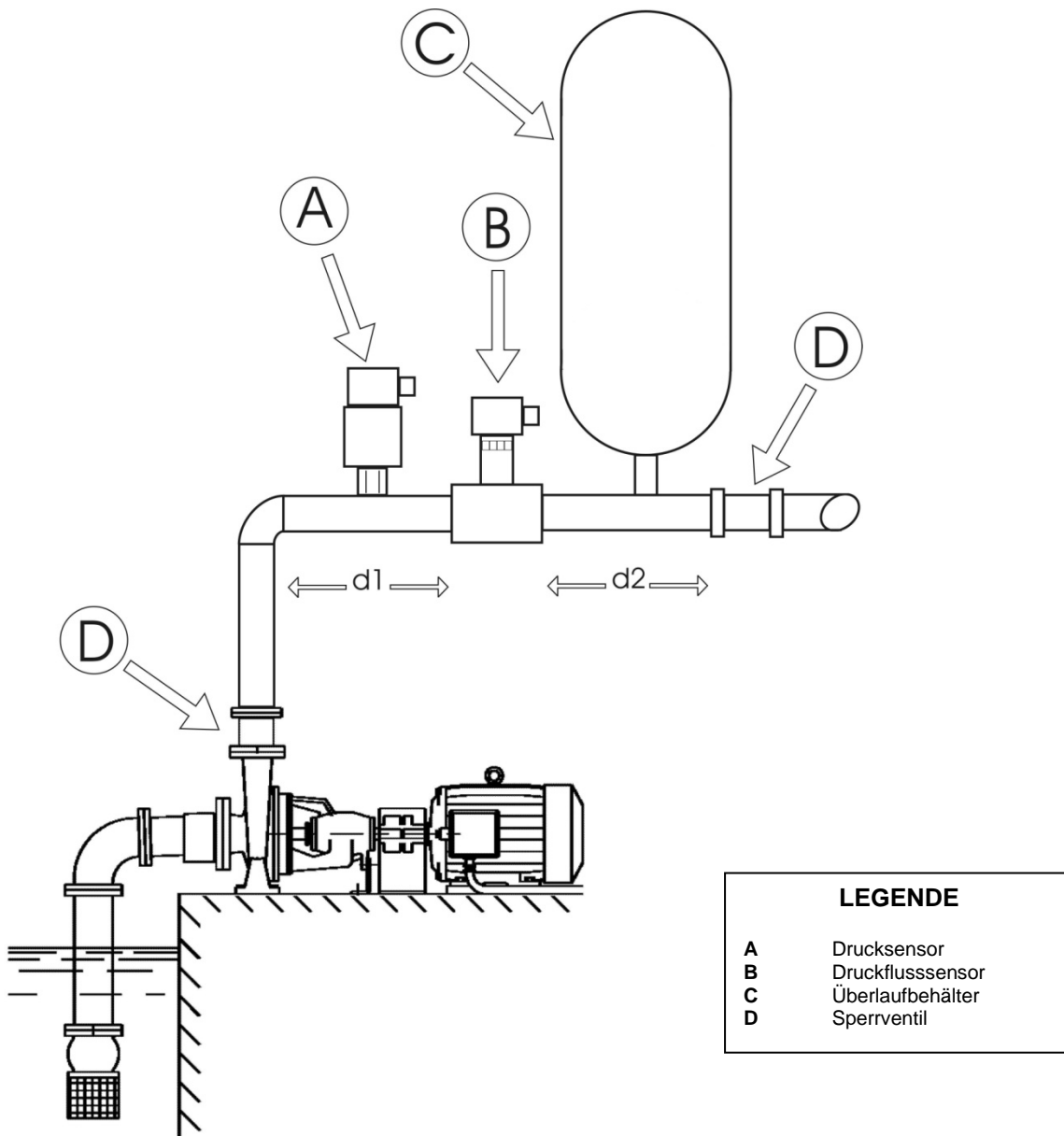
Abbildung 6: Hydraulik-Installation
