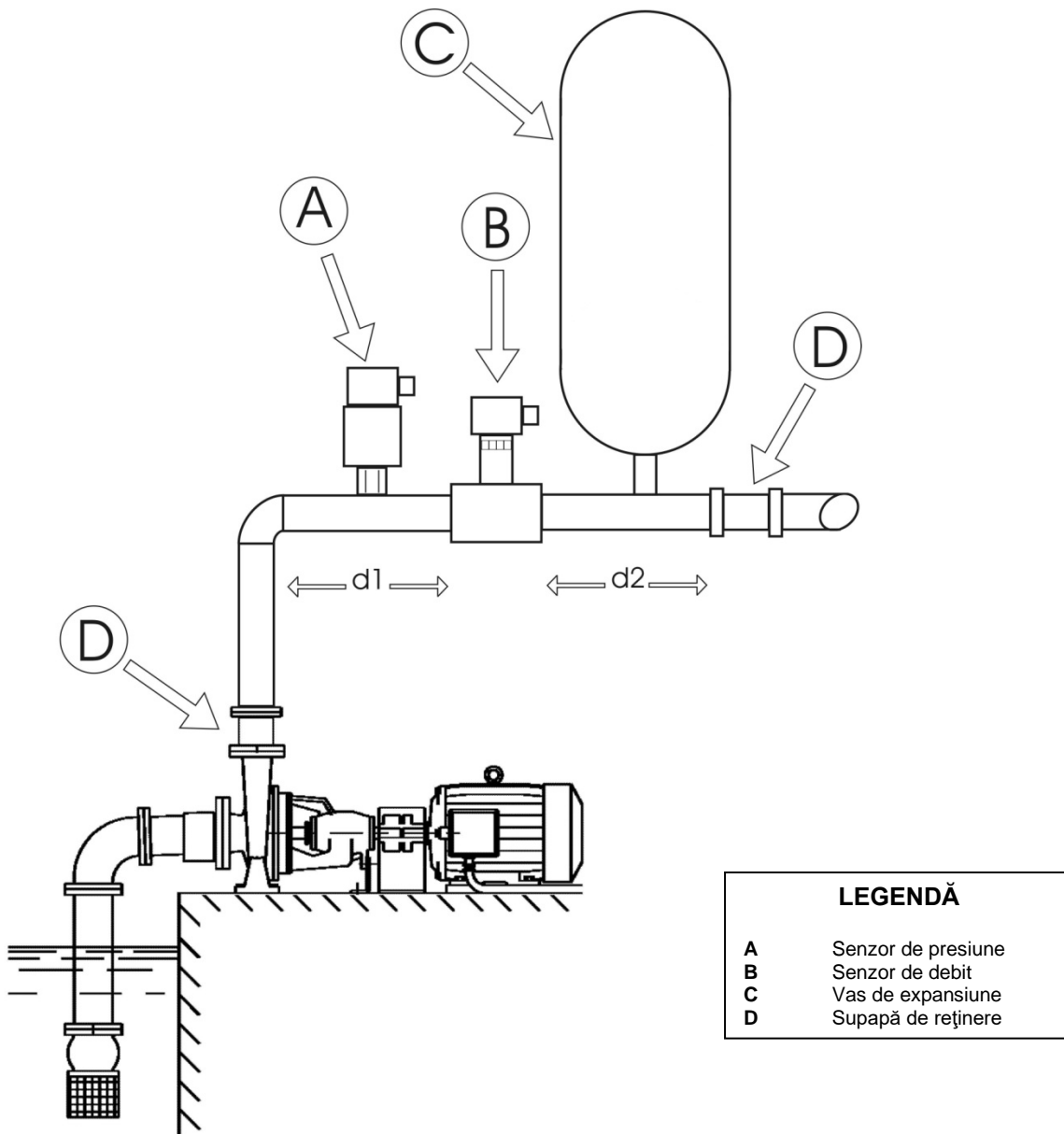
Figura 6: Instalația hidraulică
