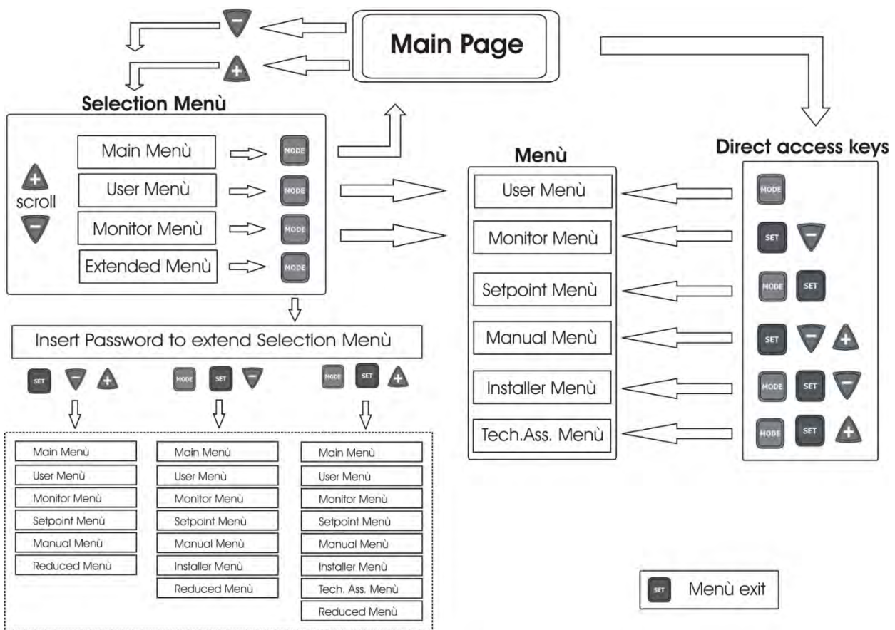
Fig. 14: Schema över menyåtkomst
