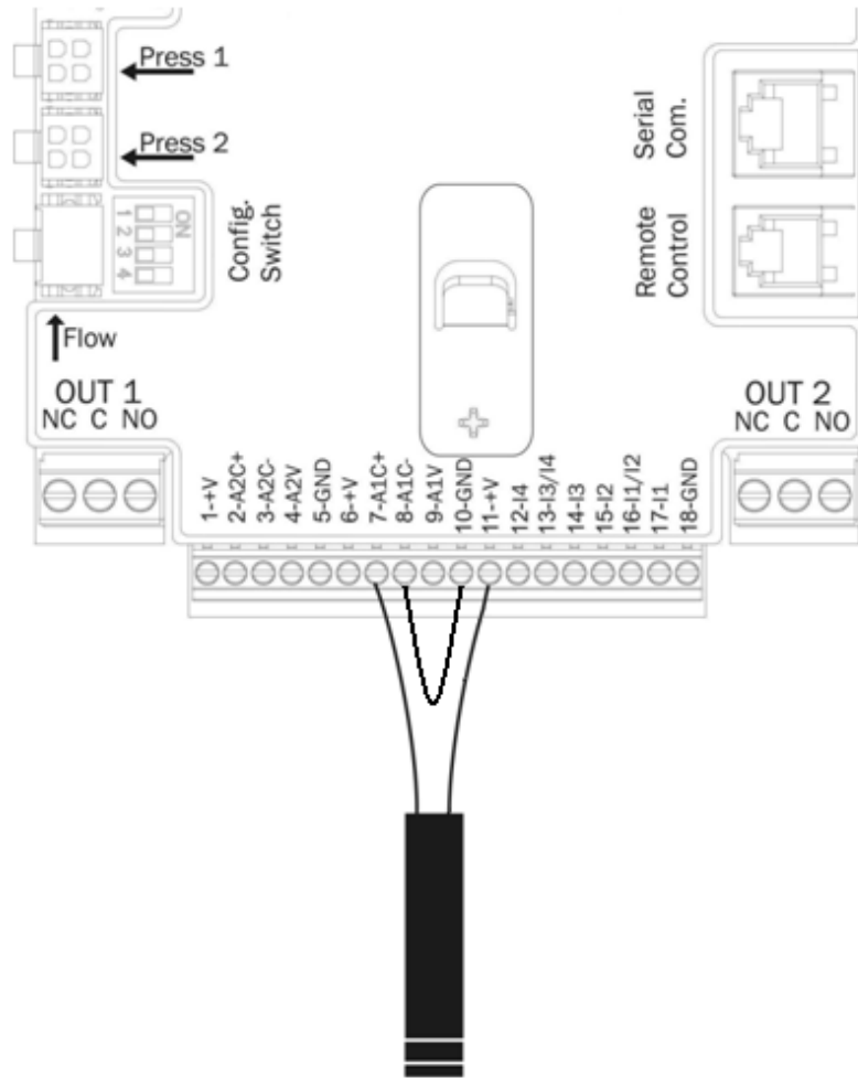
Σχήμα 8: Σύνδεση αισθητήρα πίεσης 4 - 20 mA
