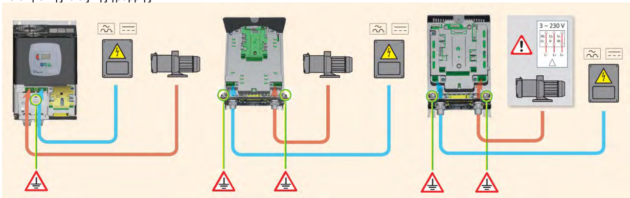
Σχήμα 4: Ηλεκτρολογικές συνδέσεις
