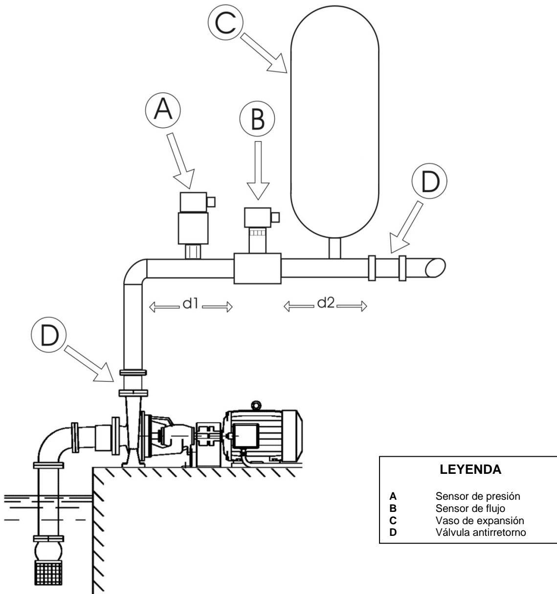
Figura 6: Instalación hidráulica
