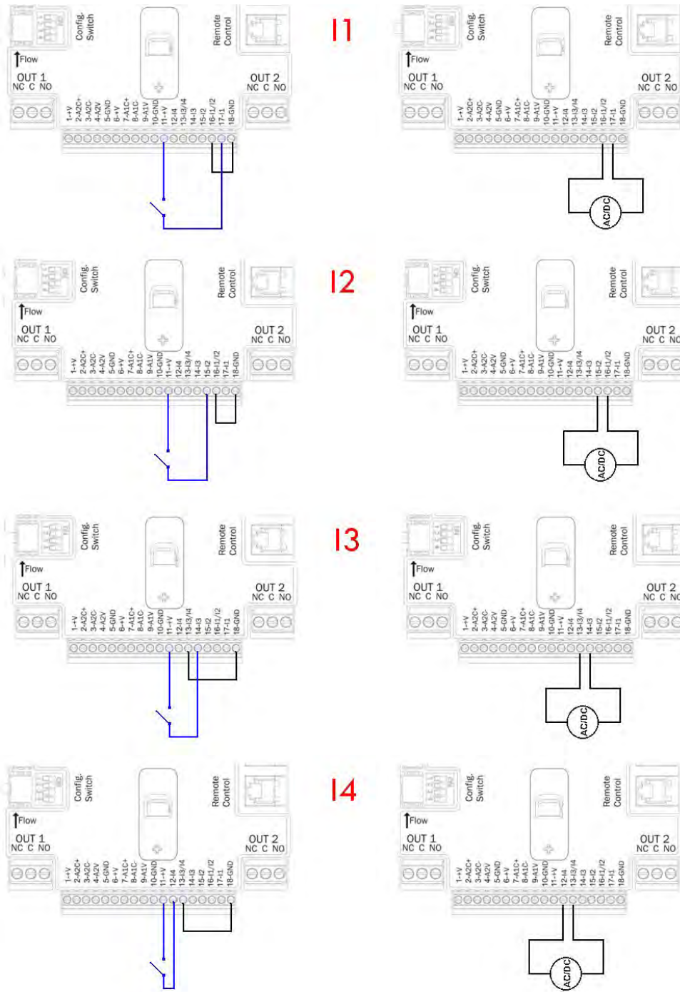
Figura 11: Esempio di collegamento degli ingressi
