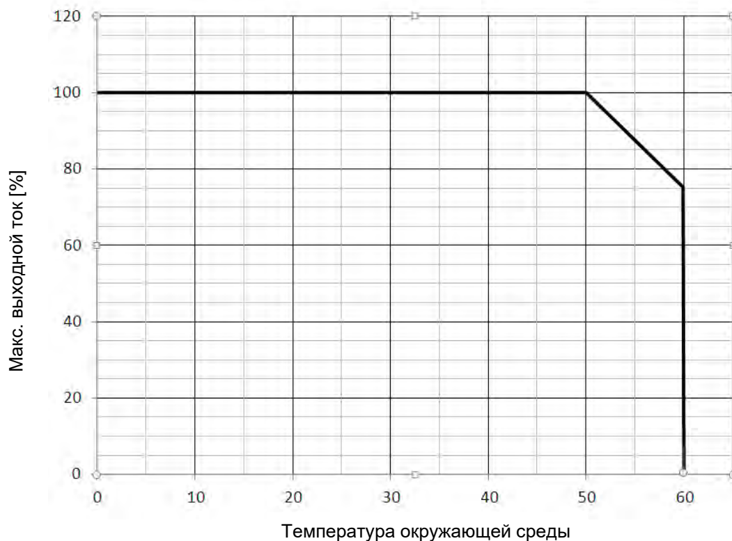
Рисунок 1: График снижения тока, в зависимости от температуры
