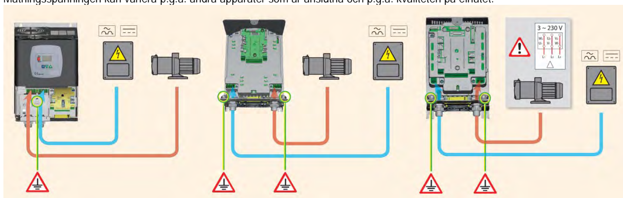
Fig. 4: Elanslutning
