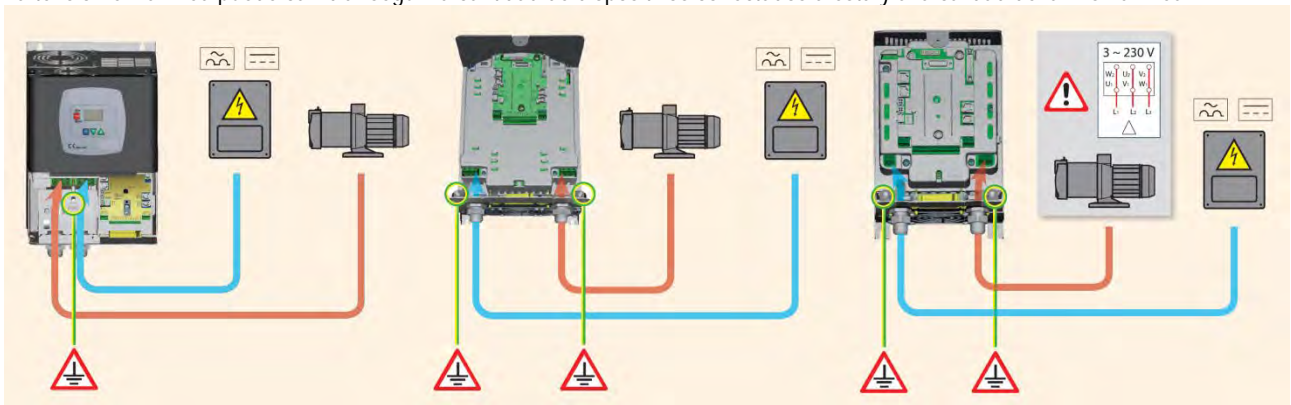
Figura 4: Conexiones eléctricas
