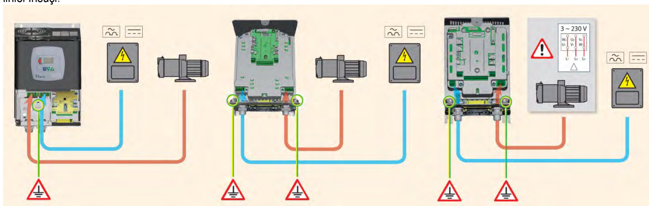
Figura 4: Conectări electrice
