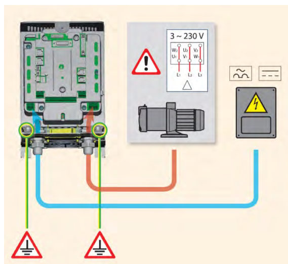
Abbildung 5: Anschluss Pumpe PWM 203 - 202 - 201
