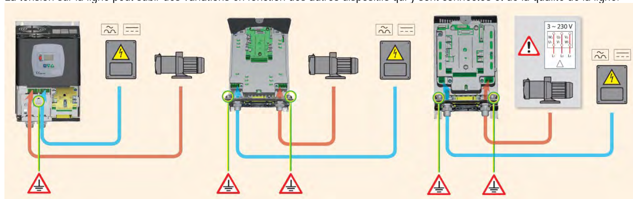
Figure 4: Connexions électriques
