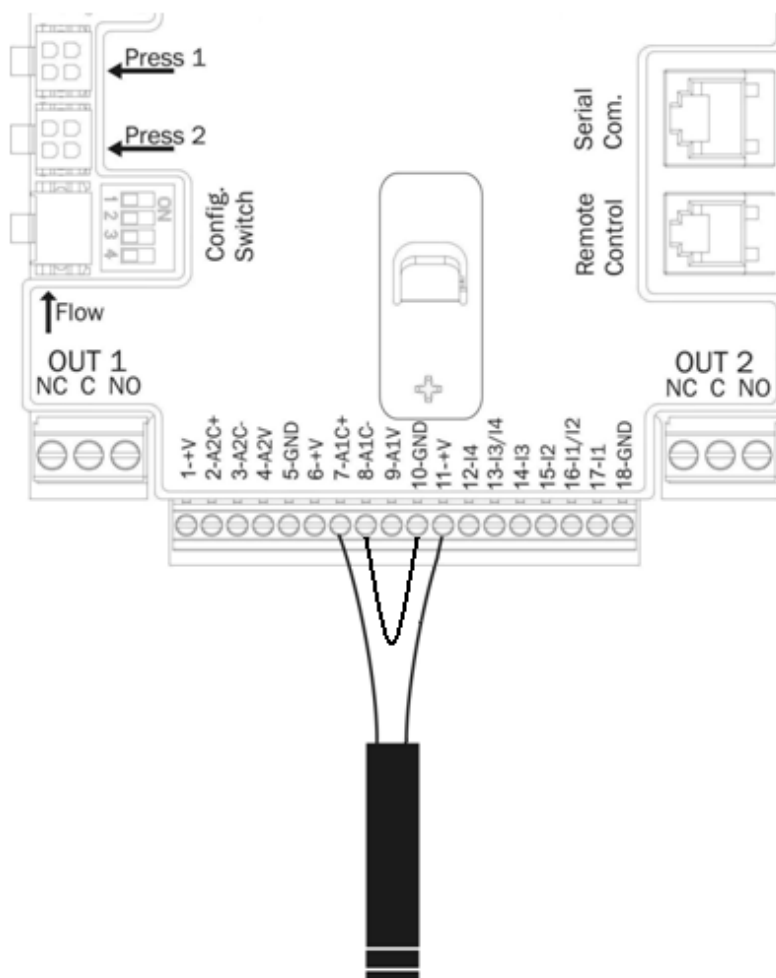
Abbildung 8: Anschluss des Drucksensors 4-20 – mA
