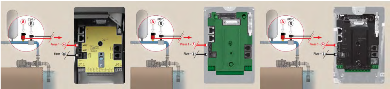
Abbildung 7: Anschluss der Sensoren
