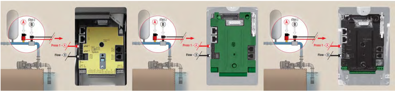
Σχήμα 7: Συνδέσεις αισθητήρων
