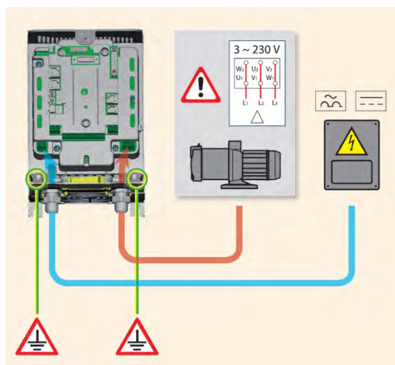
Afbeelding 5: Aansluiting pomp PWM 203 - 202 - 201
