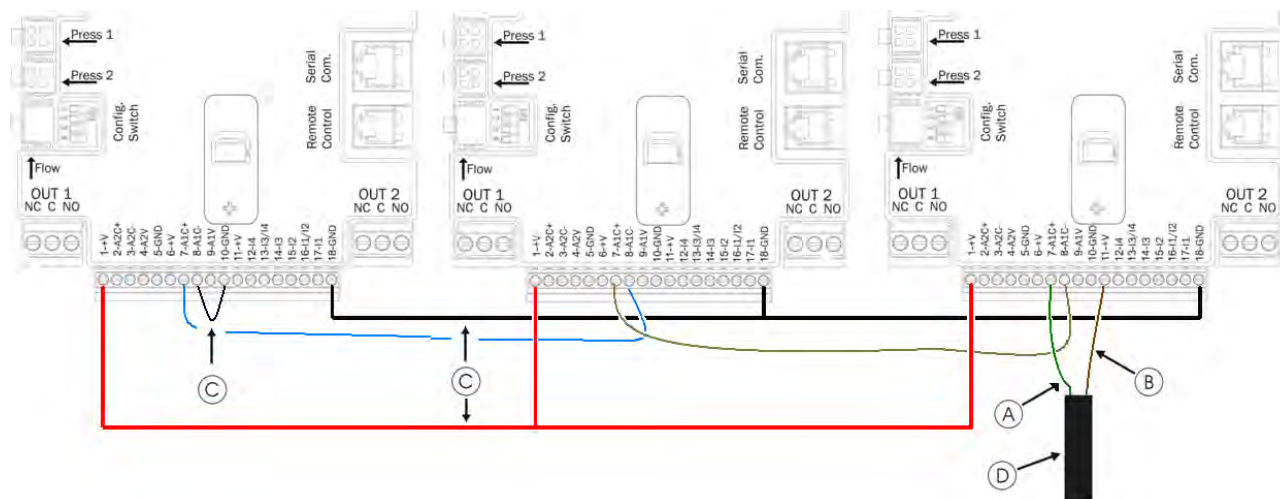
Fig. 9: Anslutning av trycksensor 4 - 20 mA i ett system med flera invertrar
