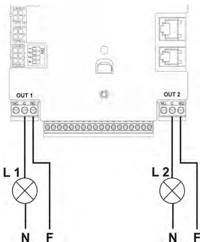
Abbildung 10: Anschlussbeispiel der Ausgänge
