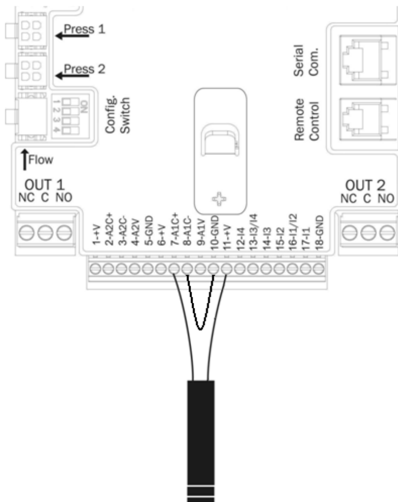
Figura 8: Collegamento sensore di pressione 4 - 20mA
