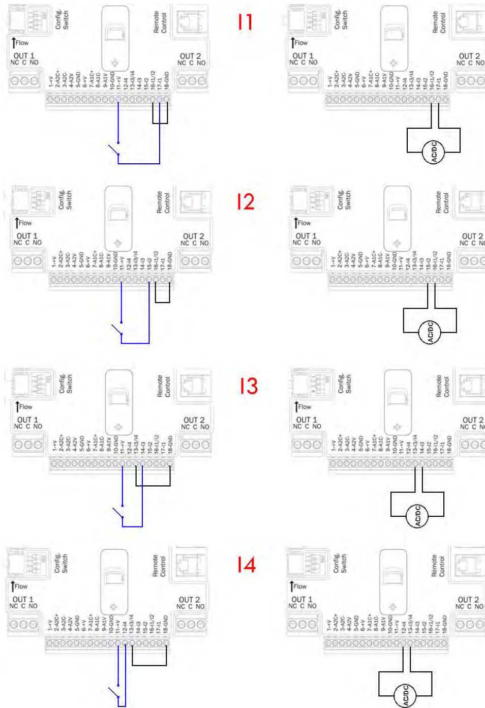
Figura 11: Ejemplo de conexión de las entradas
