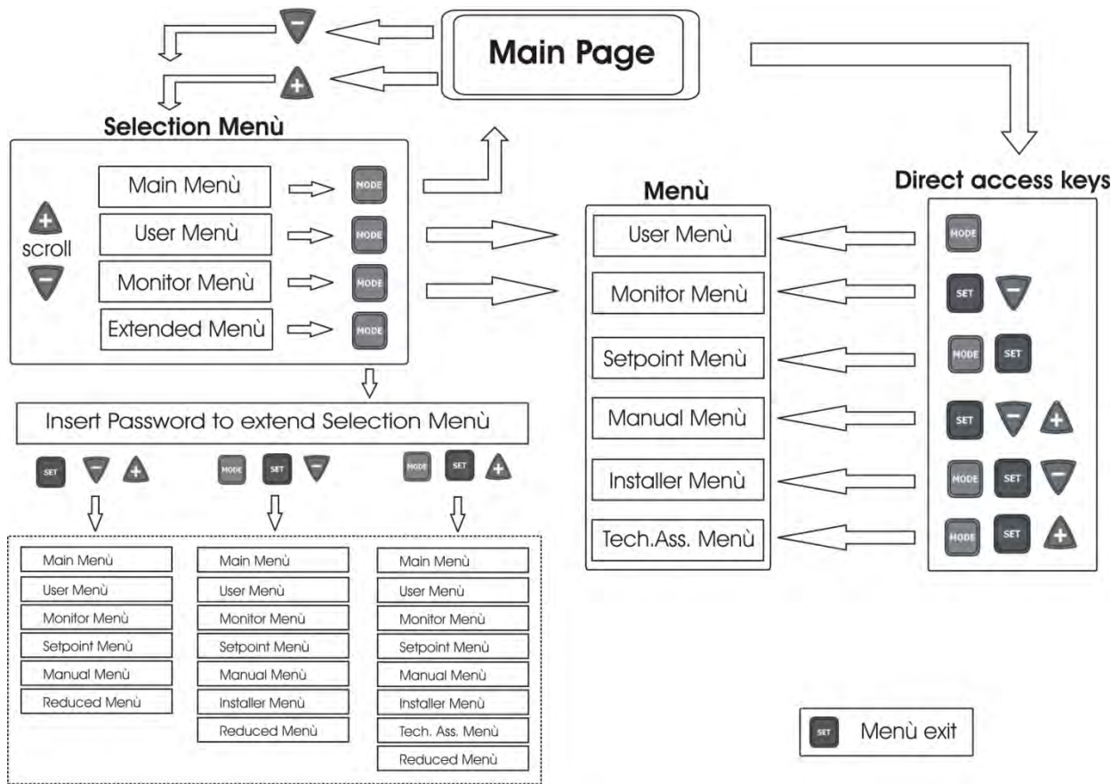
Figura 14: Schema posibilelor accesuri la meniuri
