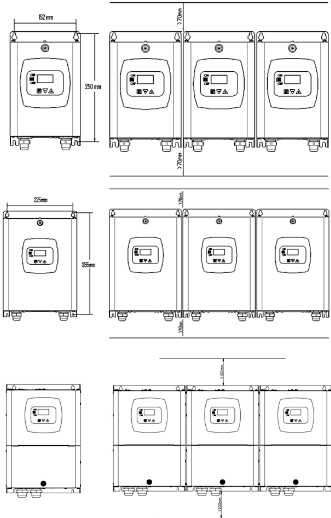
Figura 2: Fixarea și distanța minimă pentru circulația aerului
