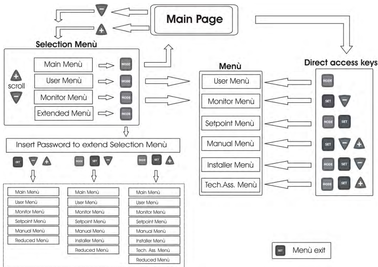
Abbildung 14: Schema der möglichen Menüzugänge
