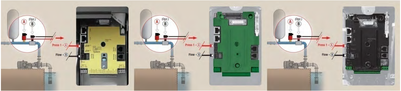
Figura 7: Connessioni sensori
