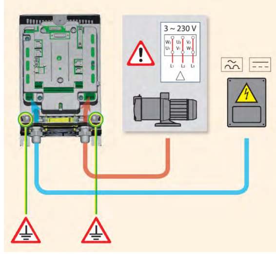
Şekil 5: PWM 203 - 202 - 201 pompa bağlantısı
