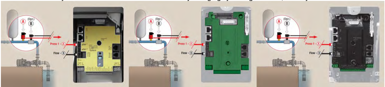
Şekil 7: Sensör bağlantıları
