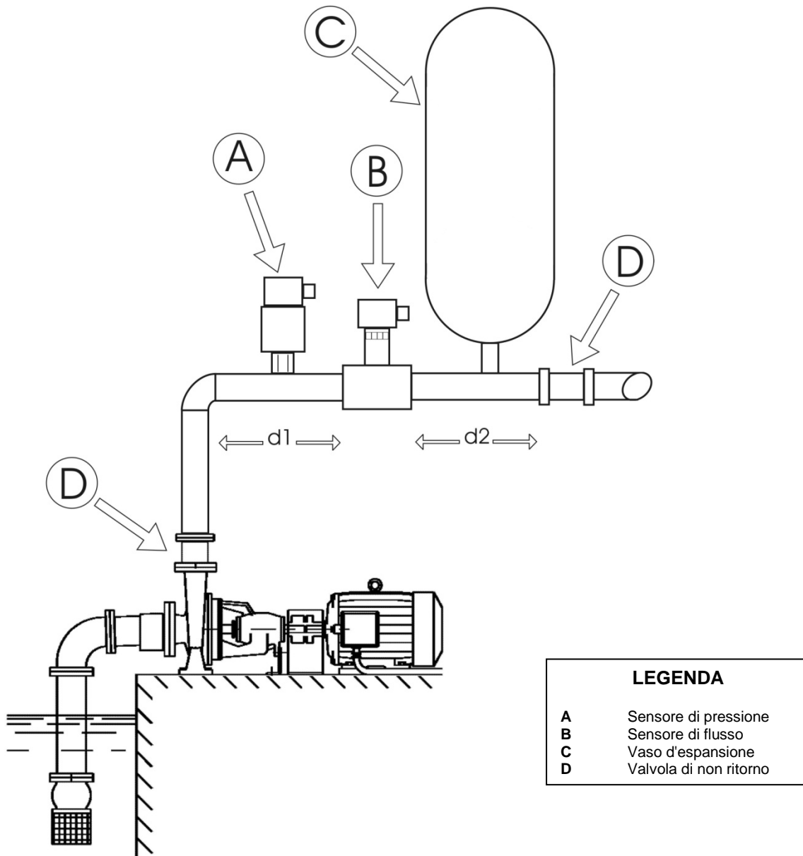
Figura 6: Installazione Idraulica
