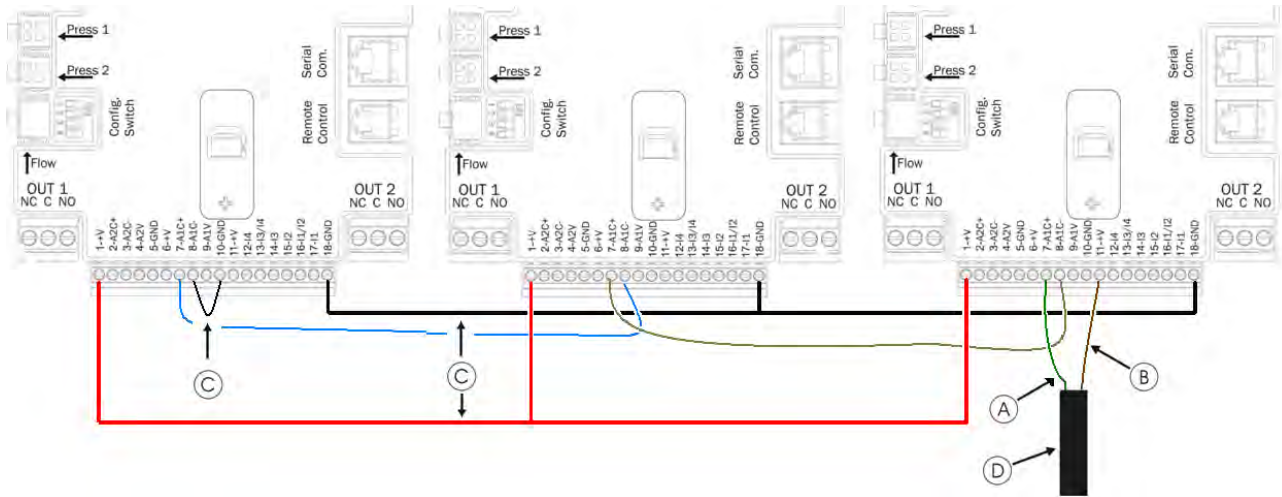
Figure 9 : Connexion capteur de pression 4 - 20 mA dans un système multiconvertisseur
