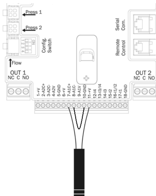
Fig. 8: Anslutning av trycksensor 4 - 20 mA
