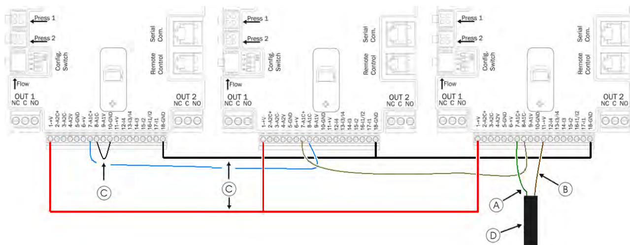
Figura 9: Conectarea senzorului de presiune 4 - 20 mA într-un sistem multi invertoare
