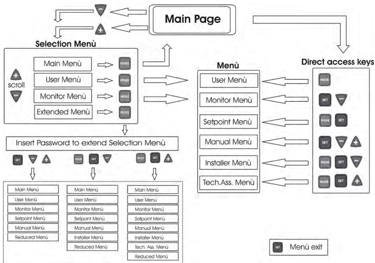
Рисунок 14: Схема различных доступов к меню
