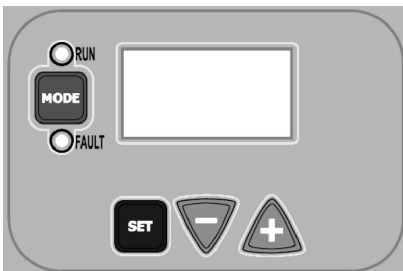
Abbildung 12: Aspekt der Nutzschnittstelle
