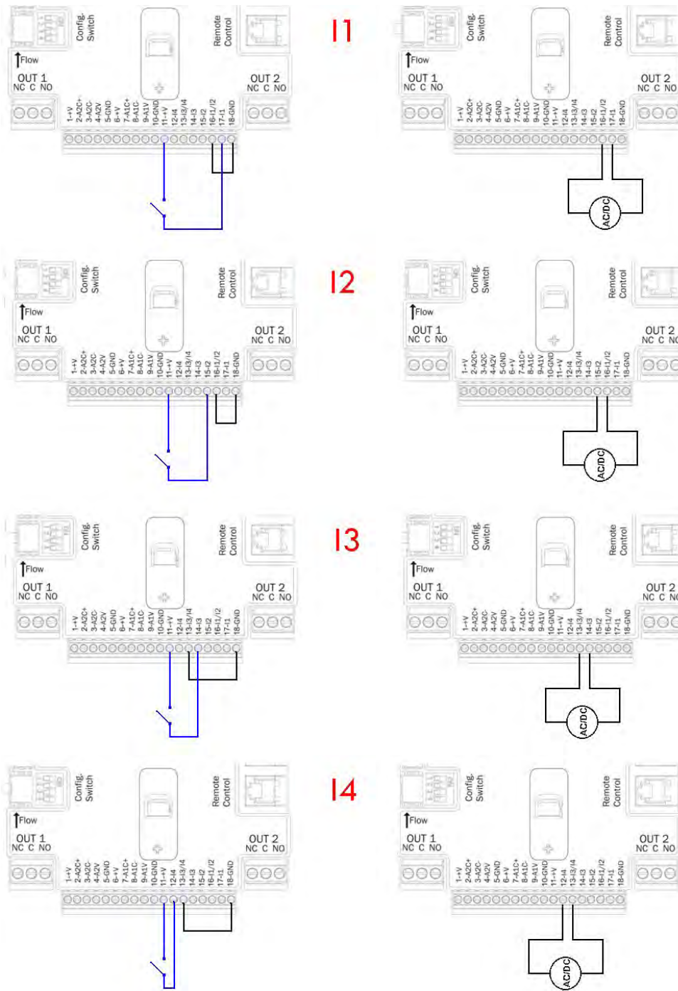
Abbildung 11: Anschlussbeispiel der Eingänge
