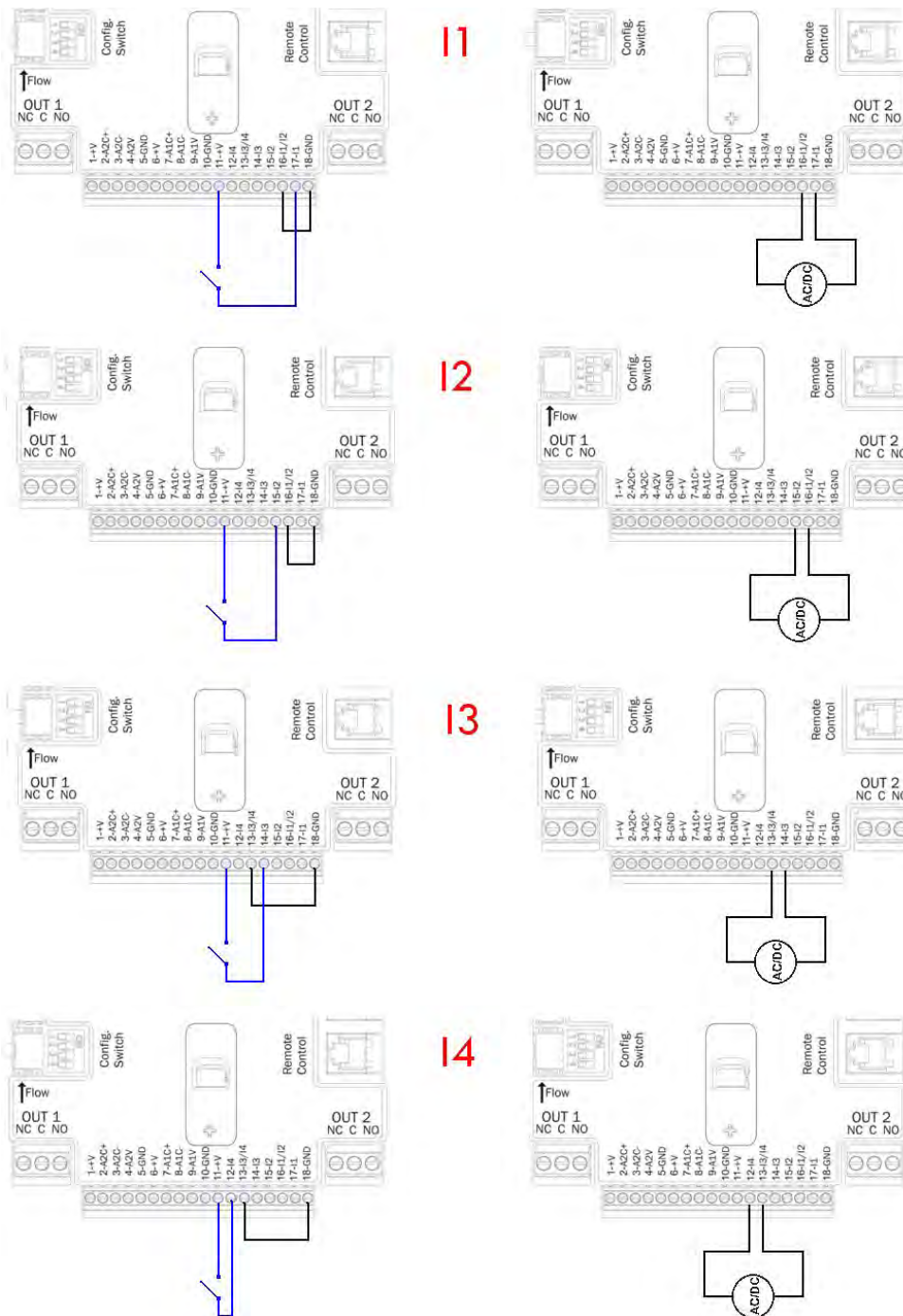
Рисунок 11: Пример соединения входов 309
