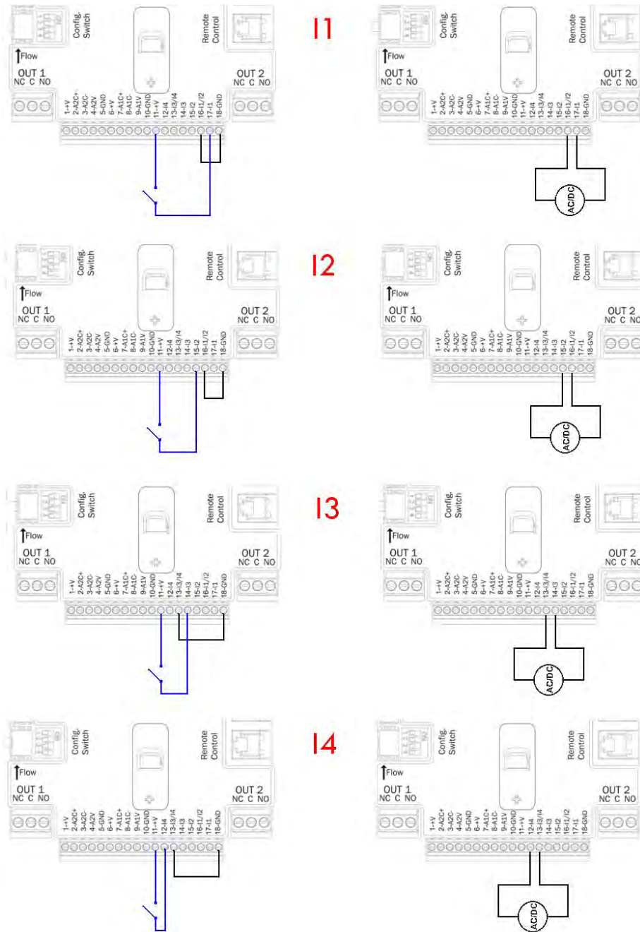
Figura 11: Exemple de conectare a intrărilor
