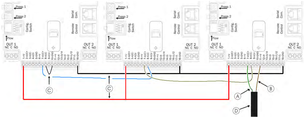
Şekil 9: 4 - 20 mA basınç sensörünün bir çoklu evirgeç sistemine bağlantısı
