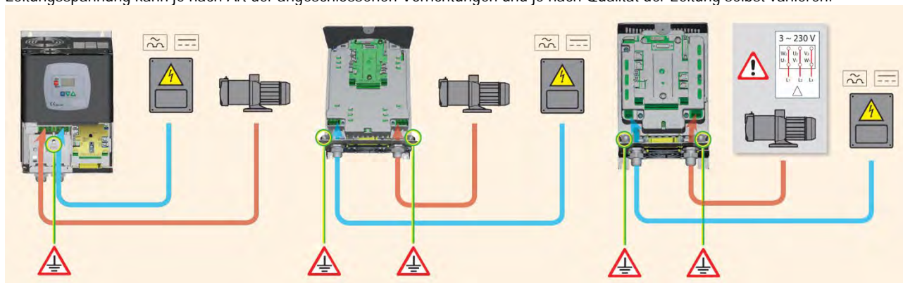
Abbildung 4: Elektrische Anschlüsse
