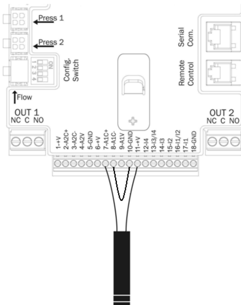
Рисунок 8: Соединение датчика давления 4 - 20 мА
