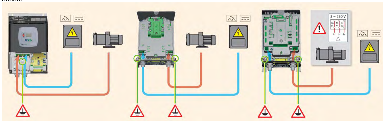
Рисунок 4: Электрические соединения
