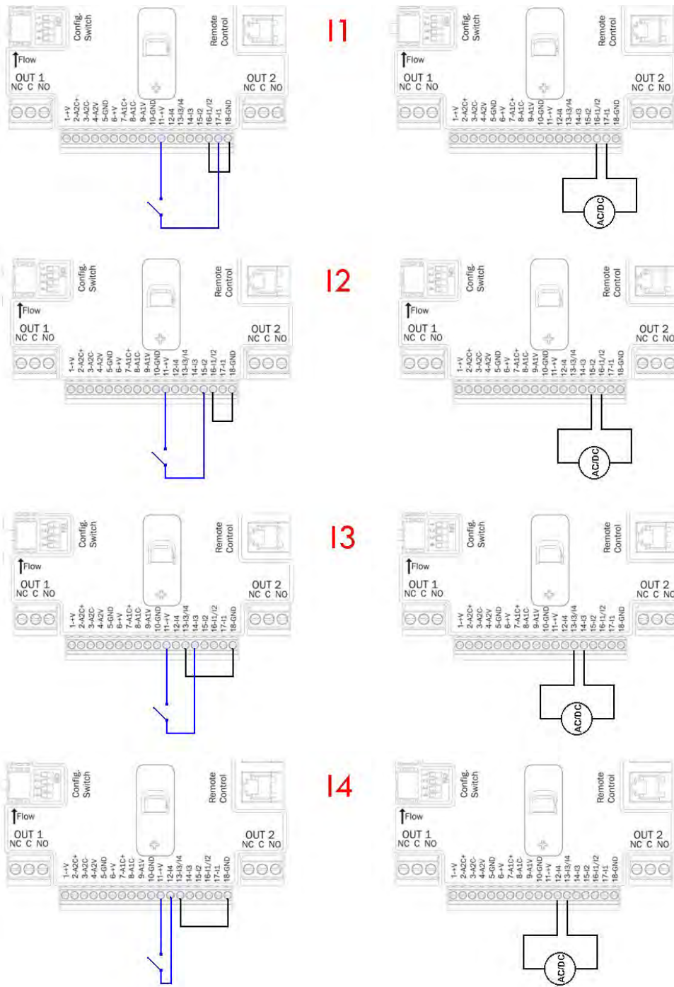
Figure11: Exemple de connexion des entrées
