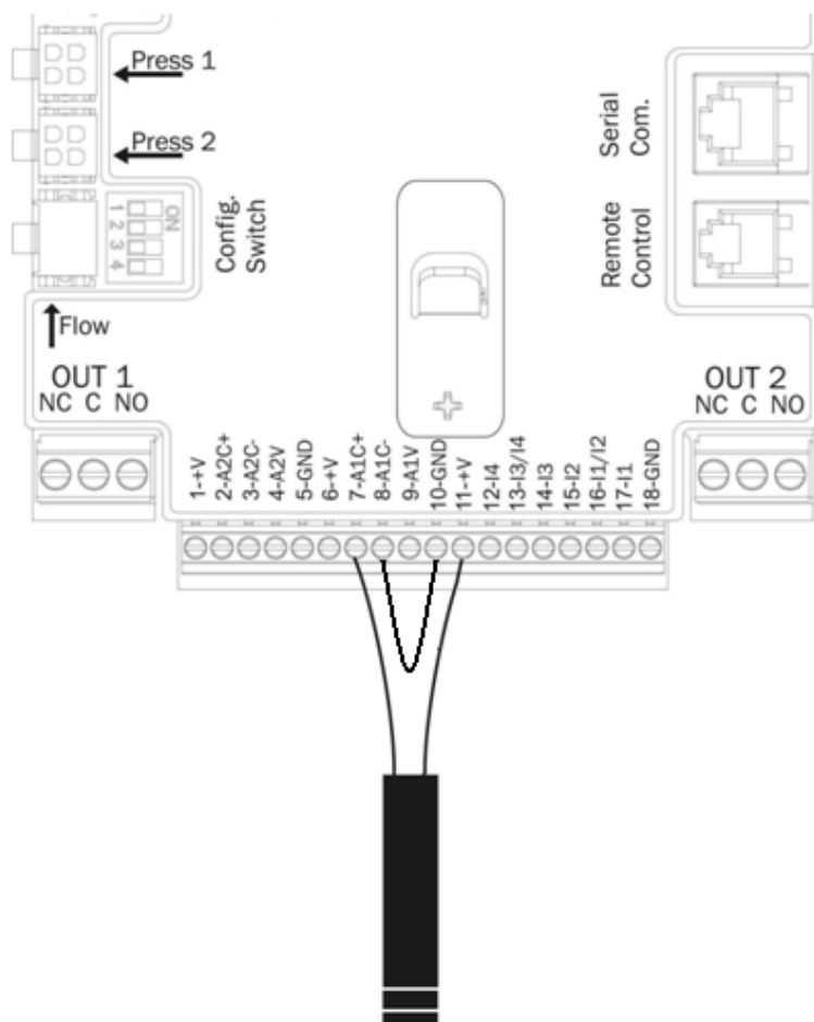
Figura 8: Conectarea senzorului de presiune 4 - 20 mA
