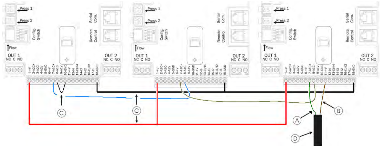
Figura 9: Conexión del sensor de presión 4 - 20 mA en un sistema multi inverter
