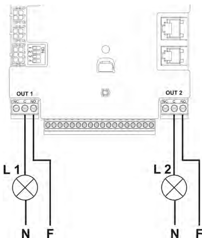
Figura 10: Esempio di collegamento delle uscite
