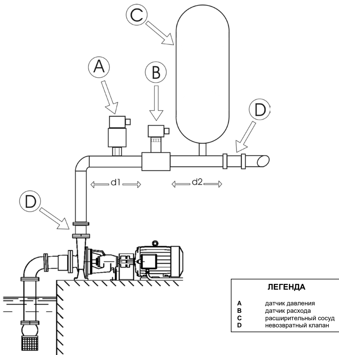
Рисунок 6: Гидравлический монтаж
