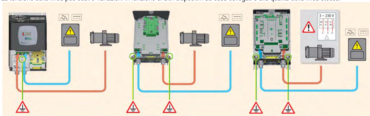
Figura 4: Connessioni elettriche
