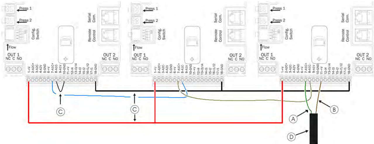
Σχήμα 9: Σύνδεση αισθητήρα πίεσης 4 – 20 mA σε ένα σύστημα multi inverter
