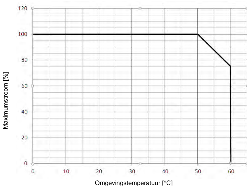
Afbeelding 1: curve stroombeperking in functie van de temperatuur
