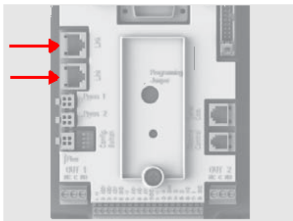
Рисунок 16: Соединение Link
