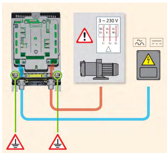
Figura 5: Collegamento pompa PWM 203 - 202 - 201
