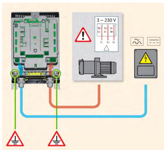
Рисунок 5: Соединение насоса PWM 203 - 202 - 201
