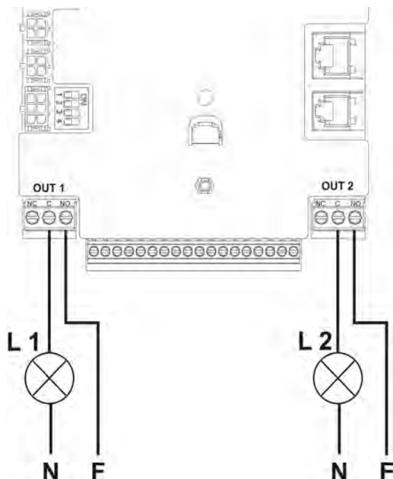
Figura 10: Ejemplo de conexión de las salidas
