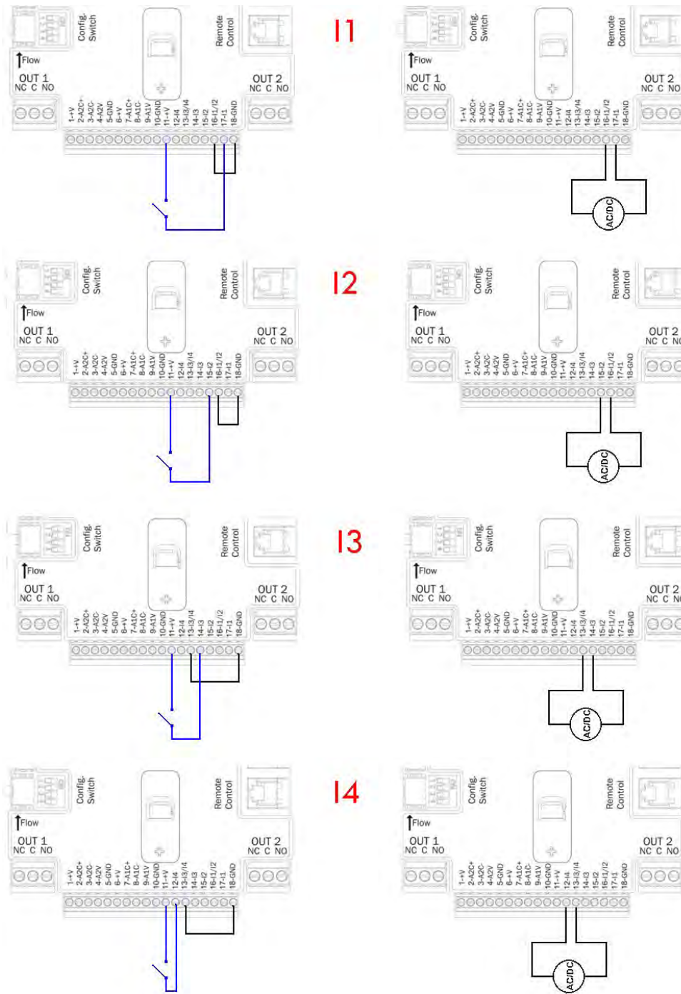
Fig. 11: Exempel på anslutning av ingångar
