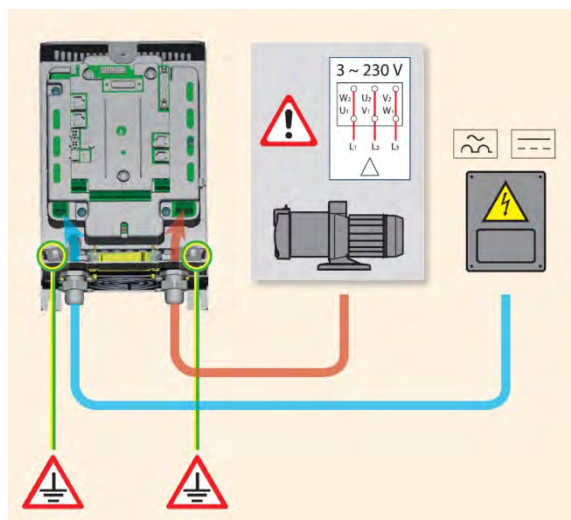
Figure 5: Connexion pompe PWM 203 - 202 - 201
