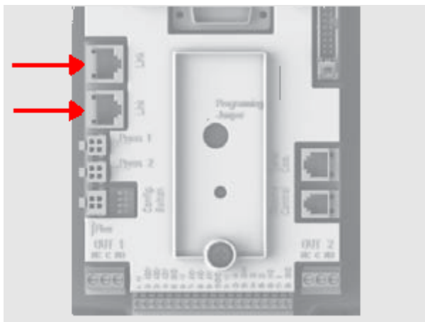
Abbildung 16: Link-Anschluss
