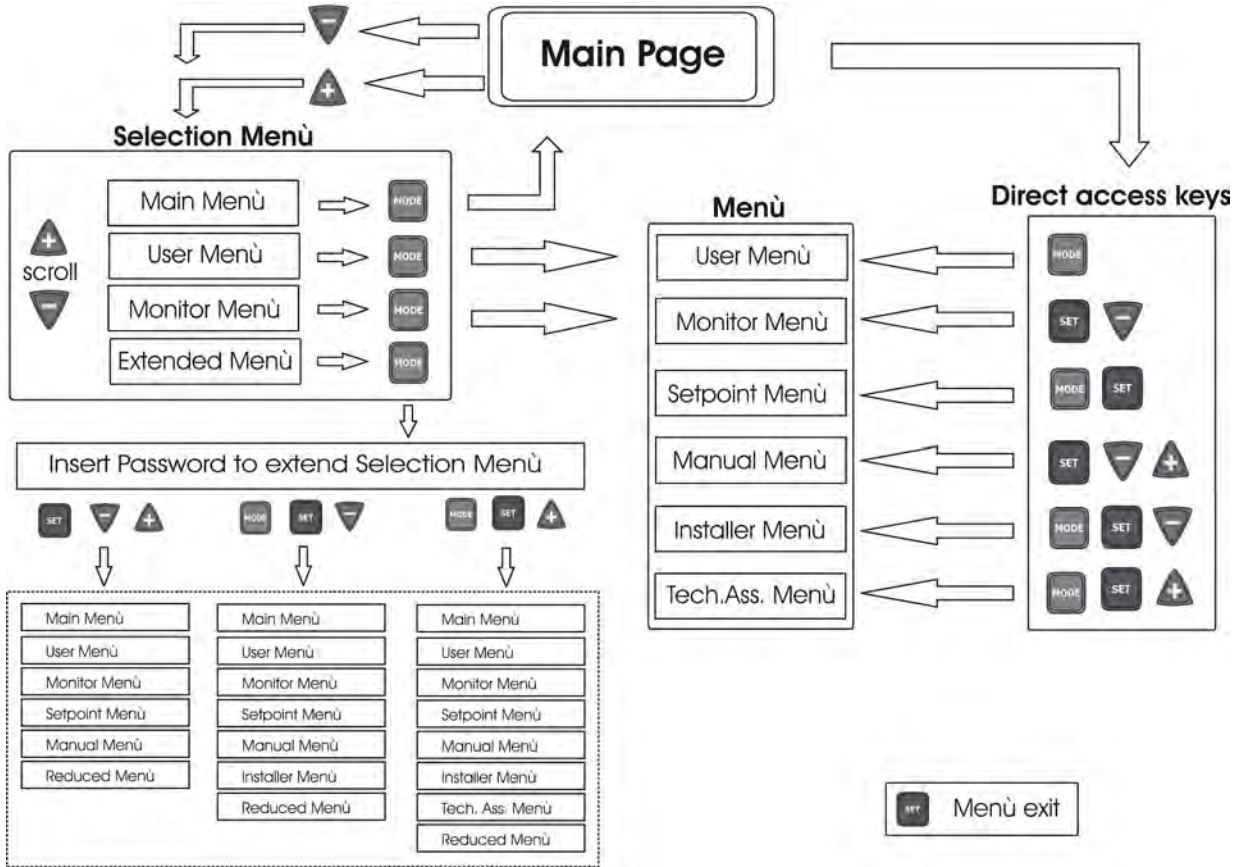
Şekil 14: İsteğe bağlı menü erişim şeması
