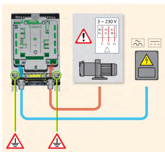
Σχήμα 5: Σύνδεση αντλίας PWM 203 - 202 - 201
