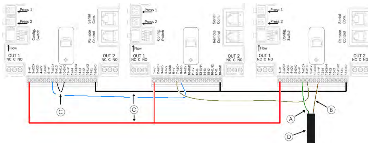
Figura 9: Collegamento sensore di pressione 4 - 20 mA in un sistema multi inverter
