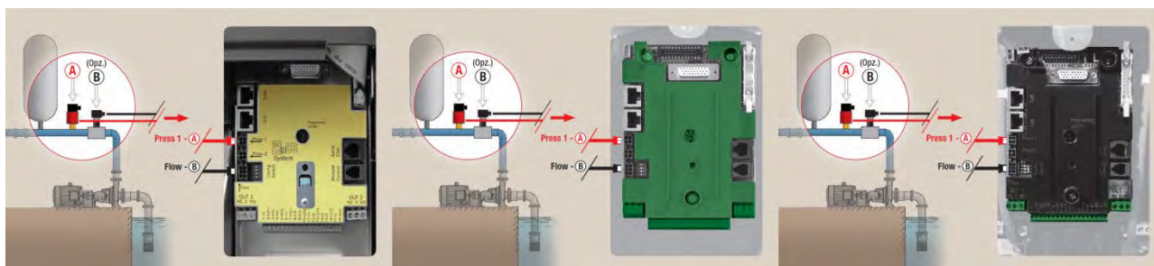
Afbeelding 7: Aansluitingen sensoren
