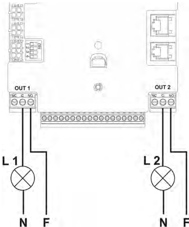
Σχήμα 10: Παράδειγμα σύνδεσης των εξόδων
