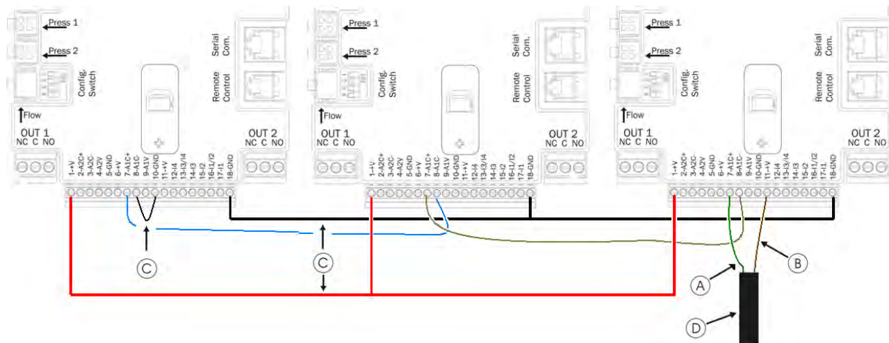
Abbildung 9: Anschluss Drucksensor 4-20 mA in einem Multi-Invertersystem
