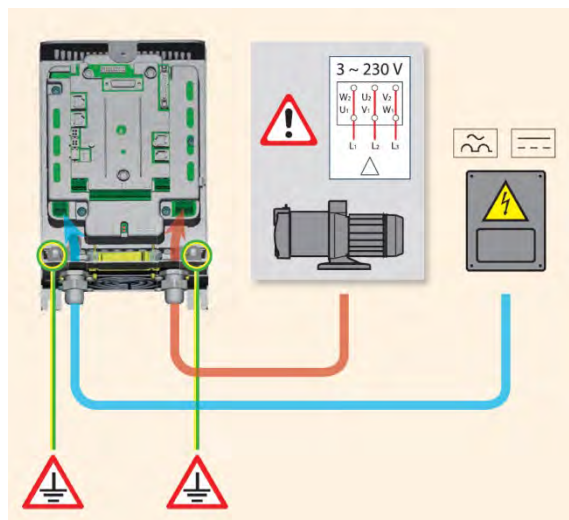
Fig. 5: Anslutning av pump PWM 203 - 202 - 201
