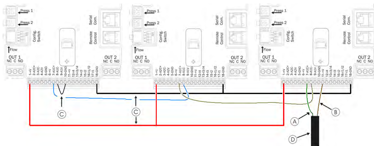
Рисунок 9: Соединение датчика давления 4 - 20 мА в системе множественных инвертеров
