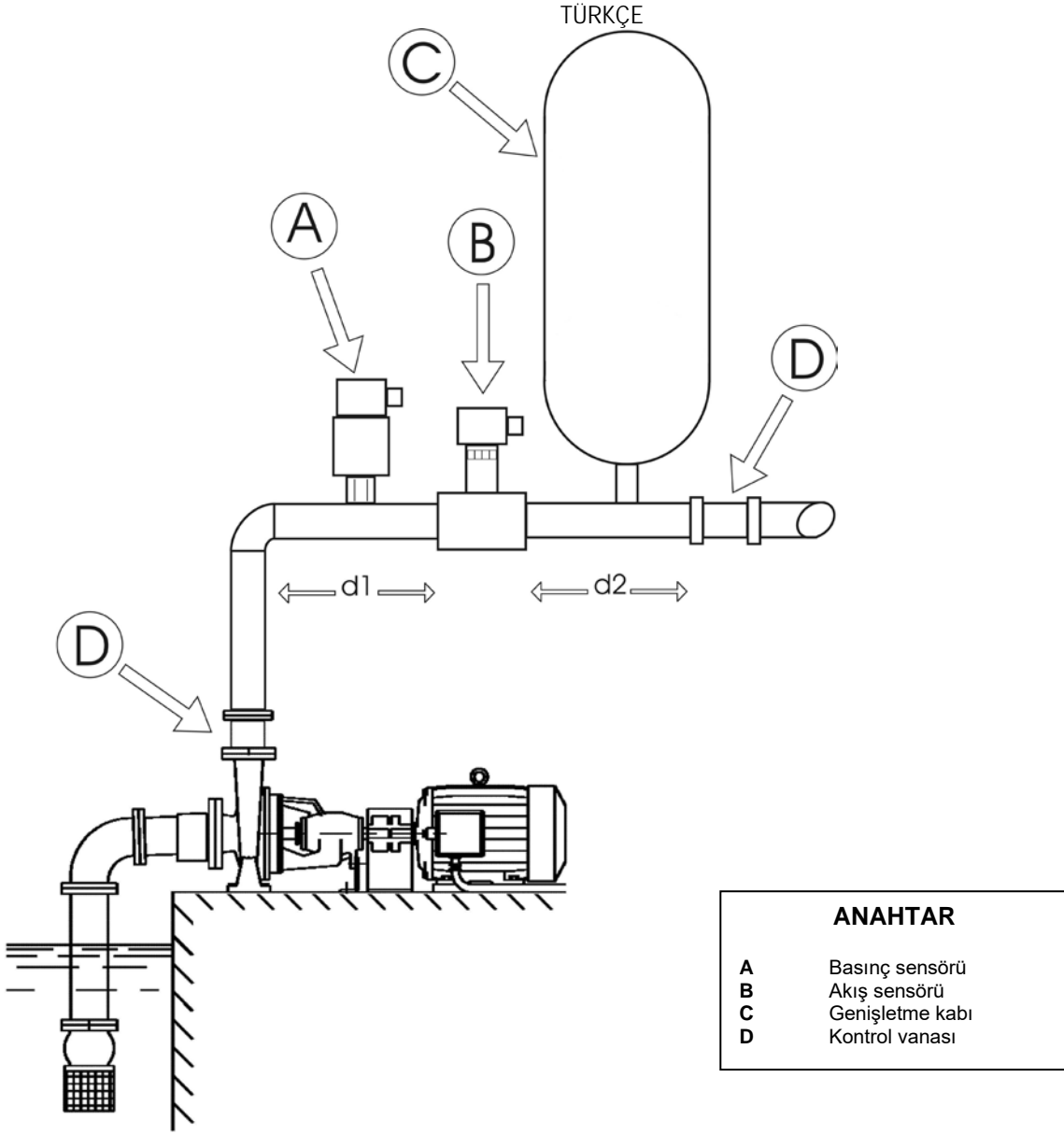
Şekil 6: Hidrolik kurulum
