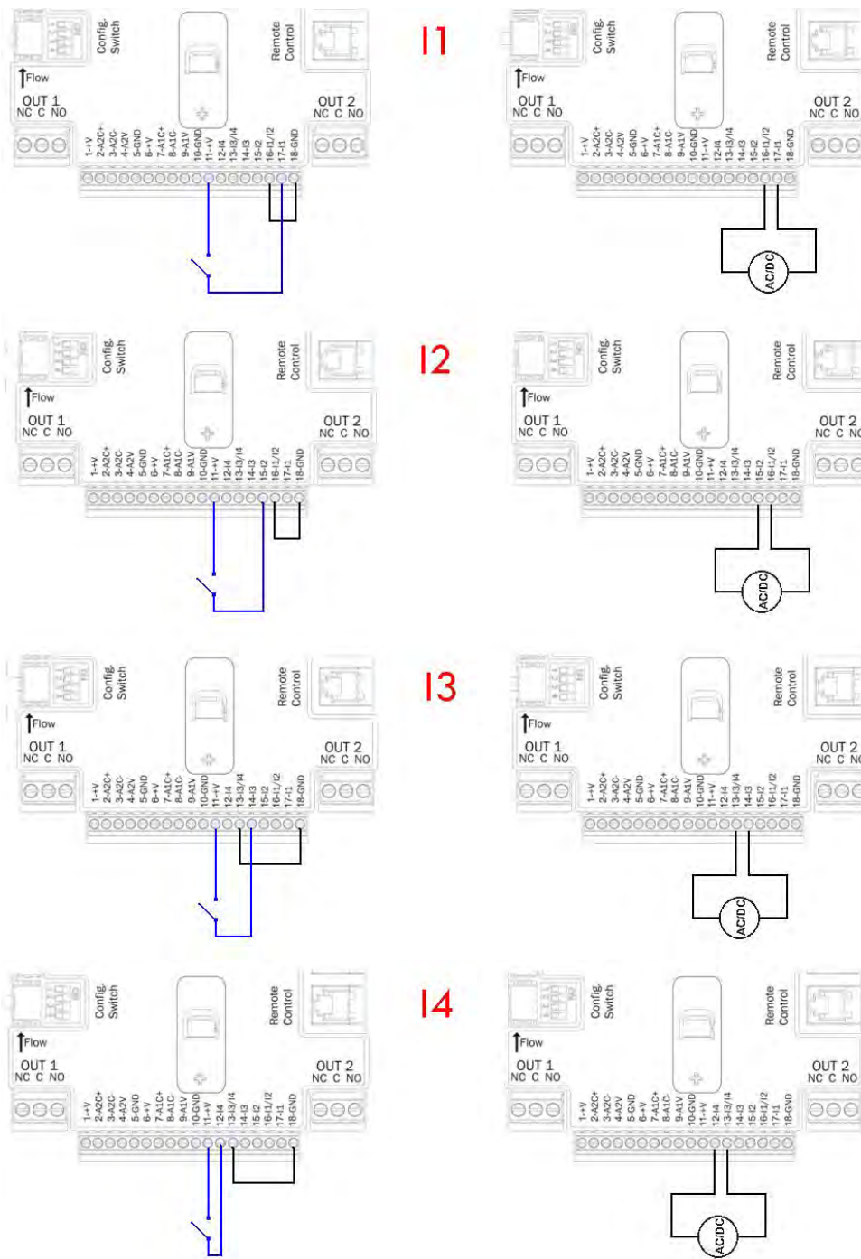
Afbeelding 11: Voorbeeld van aansluiting van de ingangen
