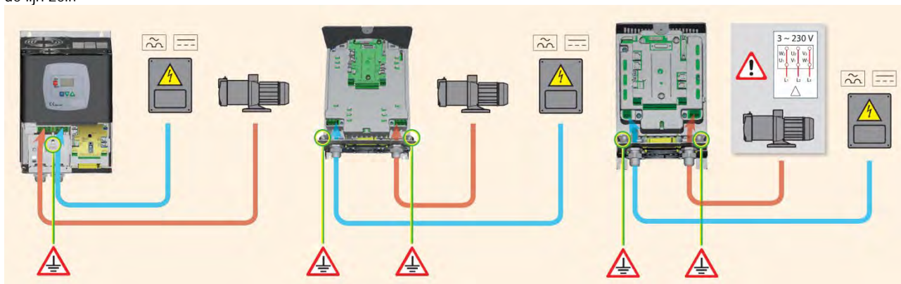
Afbeelding 4: Elektrische aansluitingen
