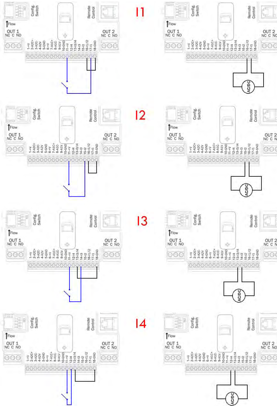
Σχήμα 11: Παράδειγμα σύνδεσης των εισόδων
