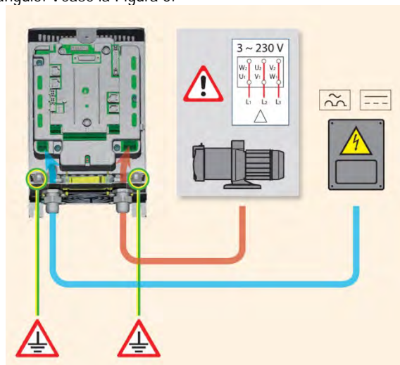
Figura 5: Conexión de la bomba PWM 203 - 202 - 201
