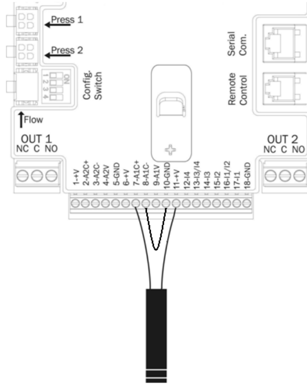
Şekil 8: 4 - 20 mA basınç sensörünü bağlama
