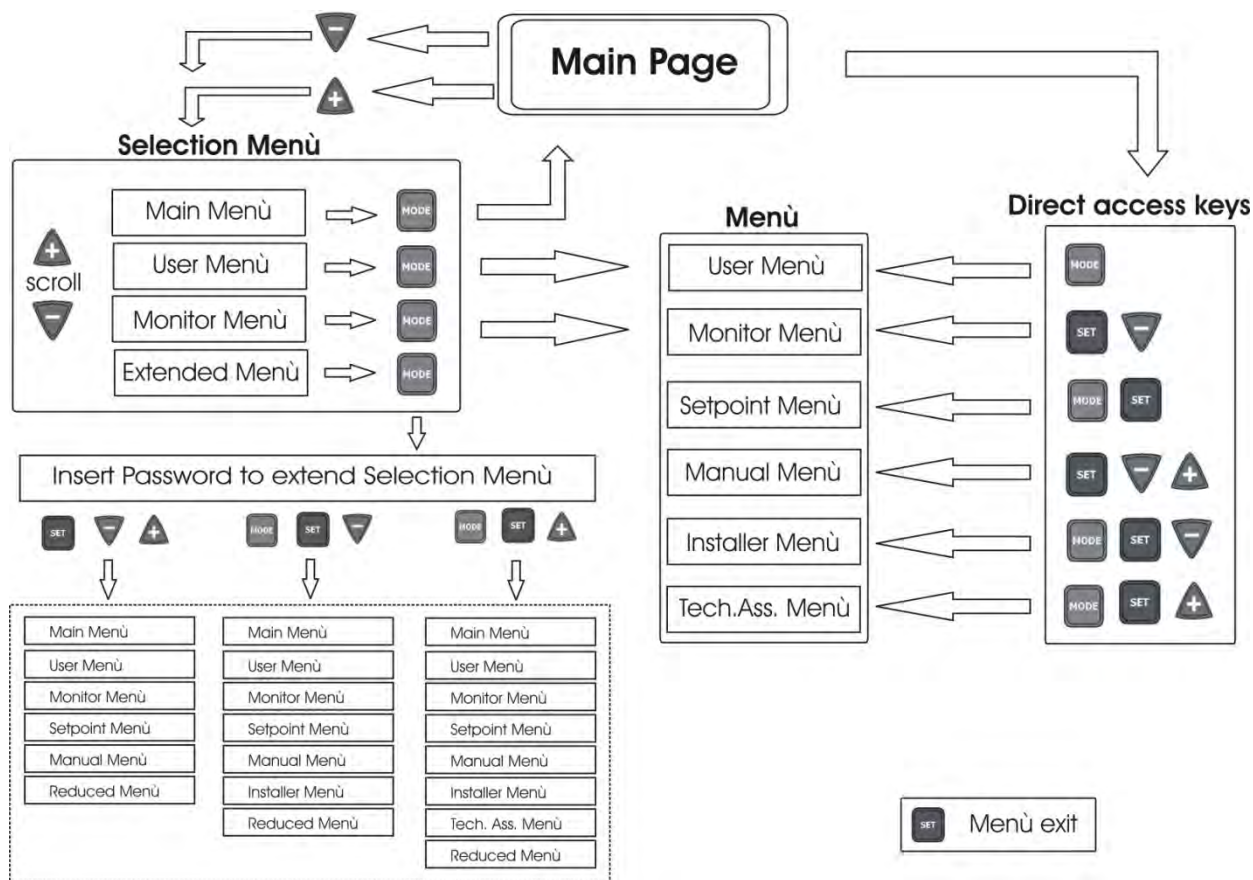
Figura 14: Schema dei possibili accessi ai menù
