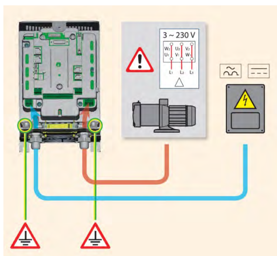
Figura 5: Conectarea pompei PWM 203 - 202 - 201
