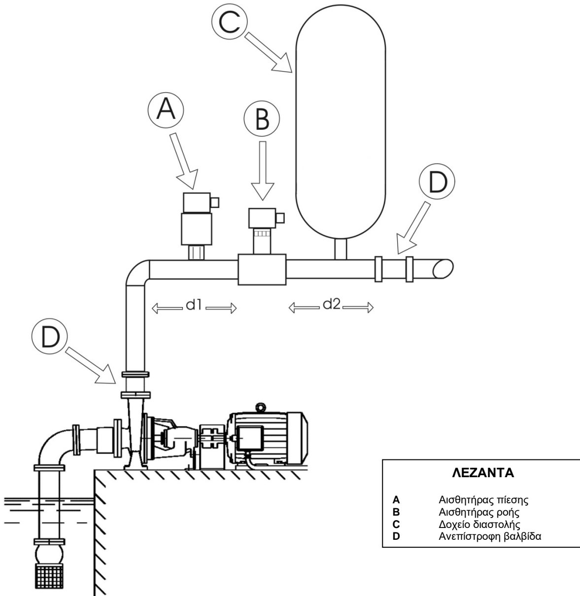
Σχήμα 6: Υδραυλική εγκατάσταση
