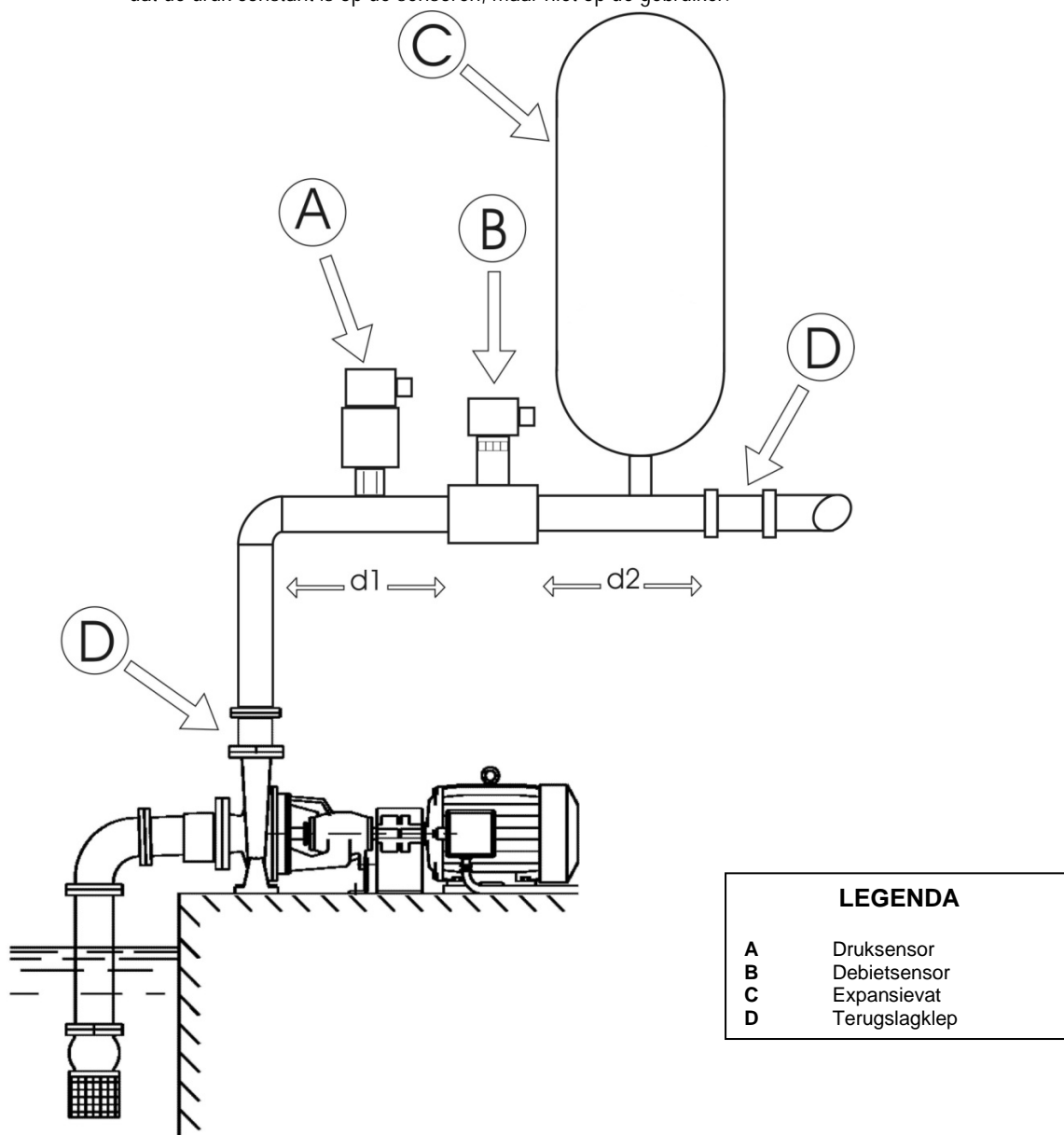
Afbeelding 6: Hydraulische installatie
