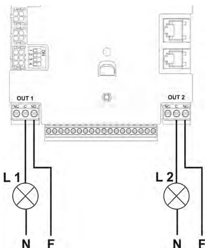
Figura 10: Exemplu de conectare a ieșirilor
