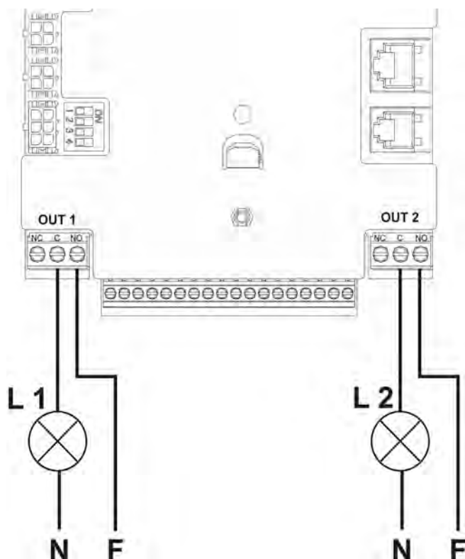
Fig. 10: Exempel på anslutning av utgångar
