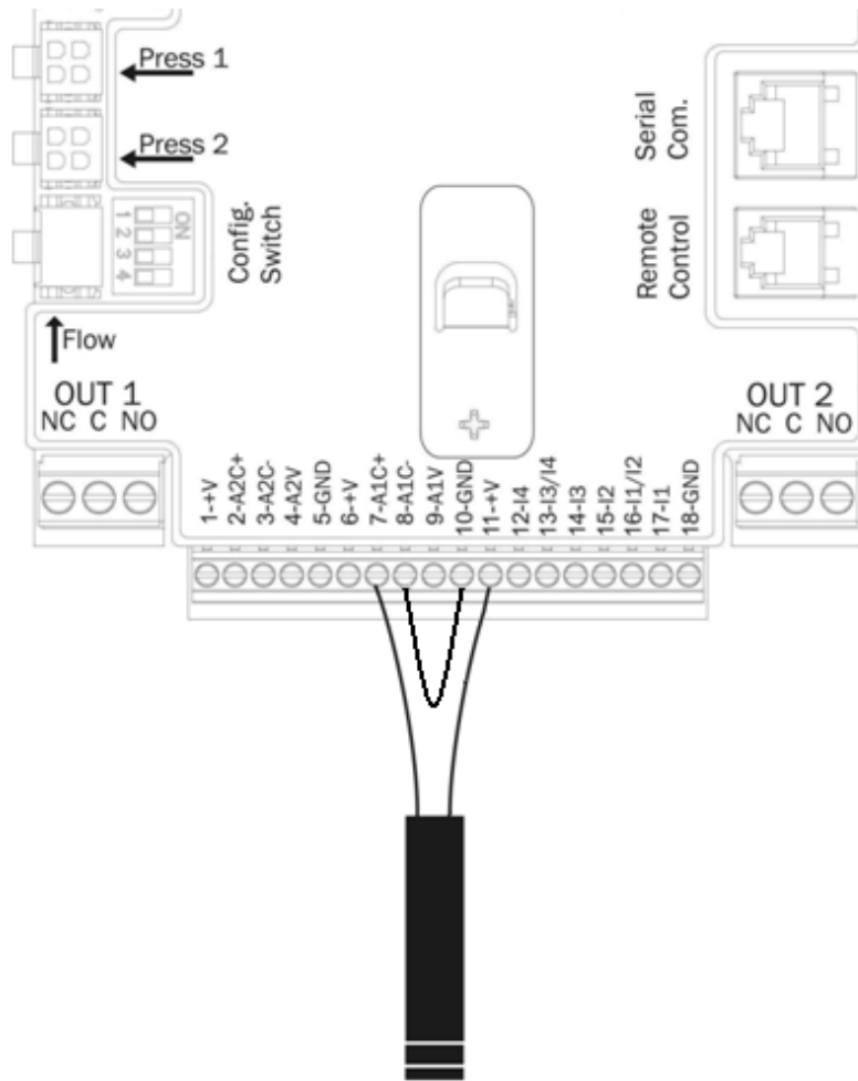
Figure 8: Connexion du capteur de pression 4 - 20 mA
