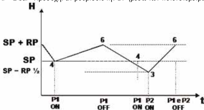
Εικόνα 17: Ρύθμιση με δοχείο διαστολής < 100 λίτρα
