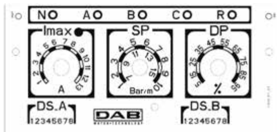
Rysunek 42: Regulacja prądu znamionowego SP i DP
