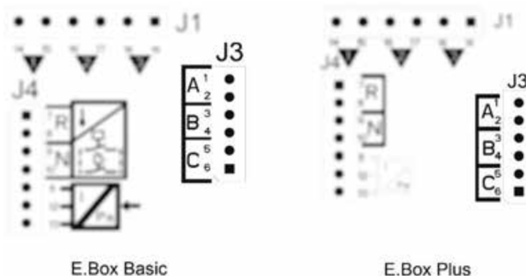
Afbeelding 47: Klemmenbord drukschakelaars
