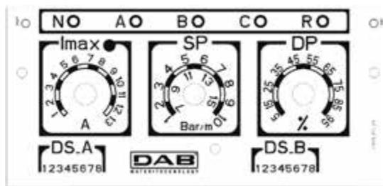
Figura 42: Regulación de la corriente nominal SP y DP
