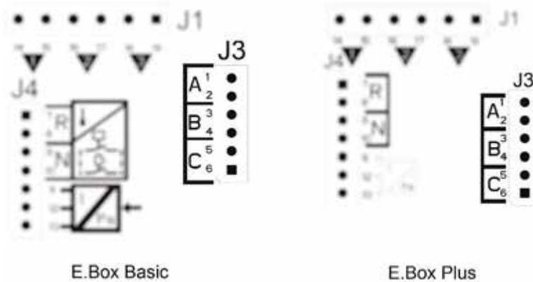
Kuva 11. Painekatkaisimien liittimet
