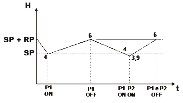
Figura 18: Regulación con vaso de expansión > 100 litros
