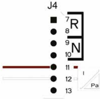
الشكل 46: توصيل مستشعر الضغط 20..4 مللي أمبير
