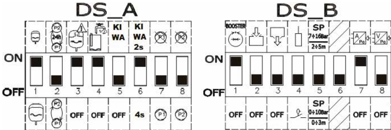
Figura 51: Interruptor DIP de presurización KIWA
