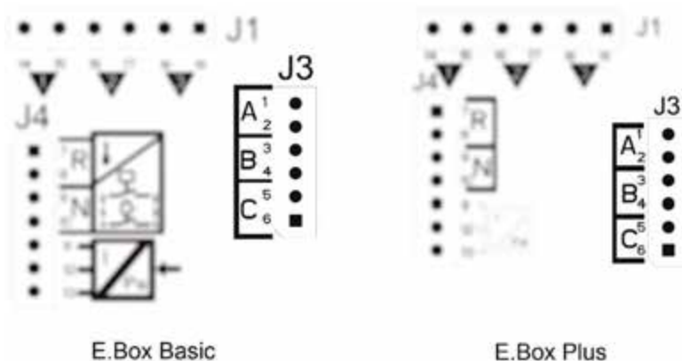
Εικόνα 47: Κλέμμα πιεσοστατών
