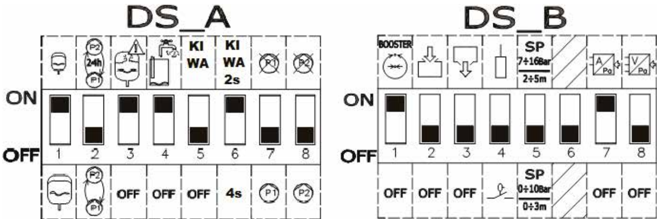
Kuva 51. Dip-kytkimet KIWA-paineistuksessa
