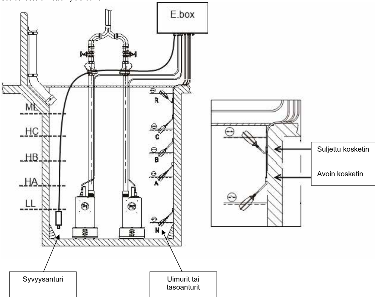
Kuva 31. Tyhjennysjärjestelmän kaavio
