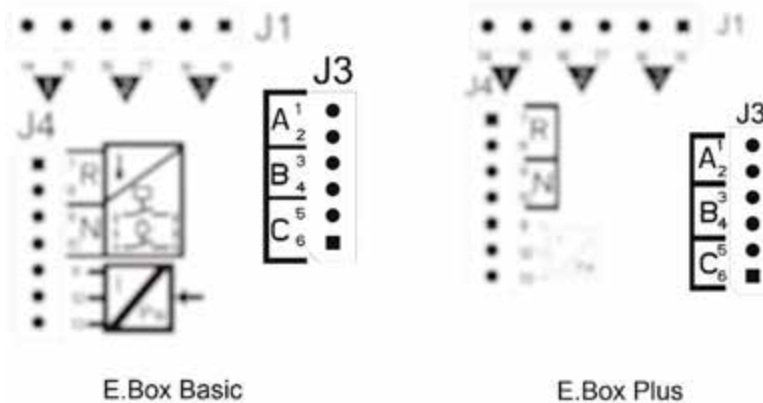
Figura 47: Borna presostați
