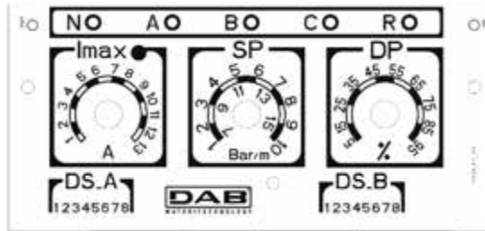
Kuva 29. SP:n ja DP:n nimellisvirran säätö
