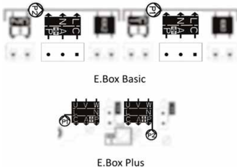
Afbeelding 3: Elektrische aansluitingen van de pompen
