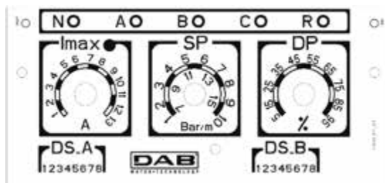
Figura 29: Regolazione corrente nominale SP e DP
