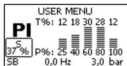
Kuva 15: tehohistogrammi
