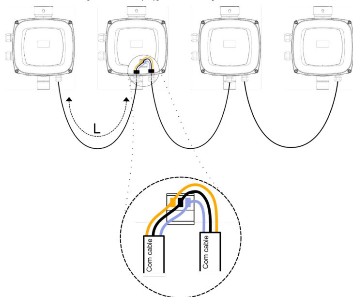
Σχήμα 6: Παράδειγμα συνδεσμολογίας της επικοινωνίας πολλαπλών αναστροφών με 4 συσκευές
