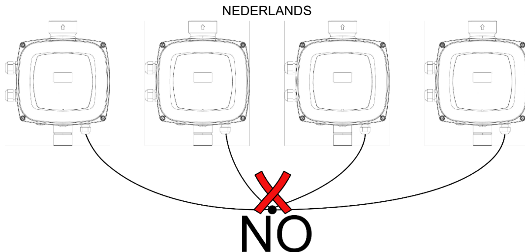
Afbeelding 8: Geen lusaansluitingen maken
