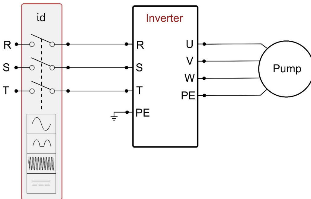
Afbeelding 3b: Installatievoorbeeld met driefasevoeding
