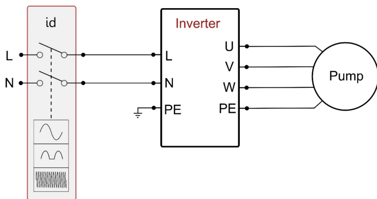
Σχήμα 2a: Παράδειγμα εγκατάστασης με μονοφασική τροφοδοσία
