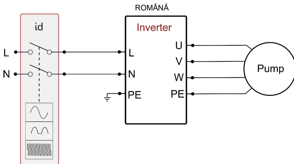
Figura 2a: Exemplu de instalare cu alimentare monofazică
