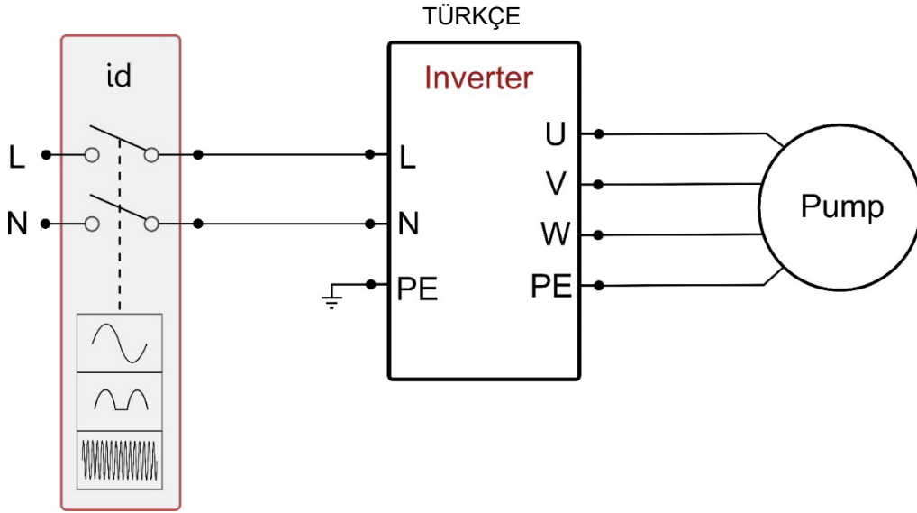
Şekil 2a: Monofaze besleme ile kurma örneğinofase
