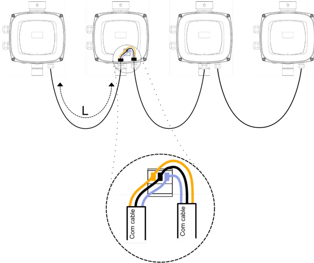
Afbeelding 6: Aansluitvoorbeeld van communicatie met meerdere inverters, met 4 apparaten
