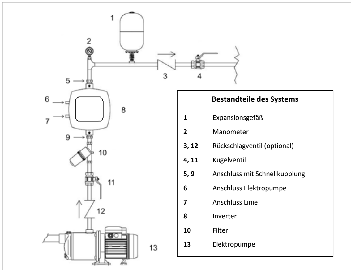
Abbildung 1: Hydraulische Installation
