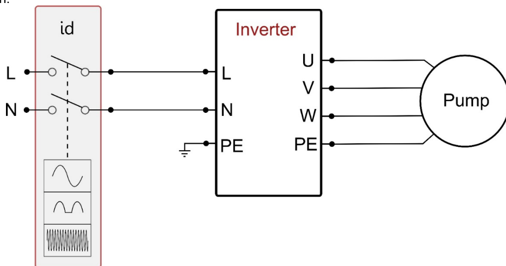
Afbeelding 2a: Installatievoorbeeld met monofasevoeding
