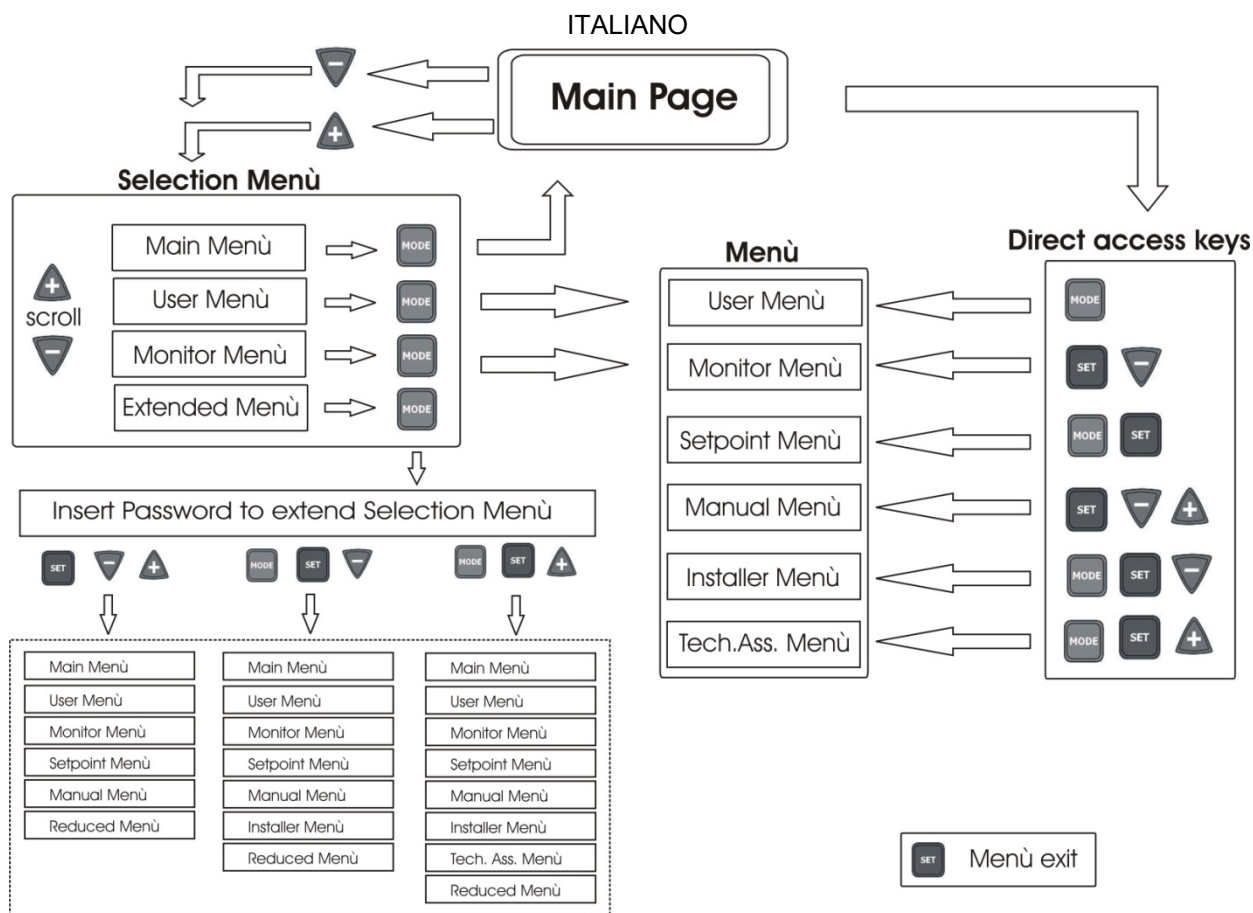
Figura 13: Schema dei possibili accessi ai menù
