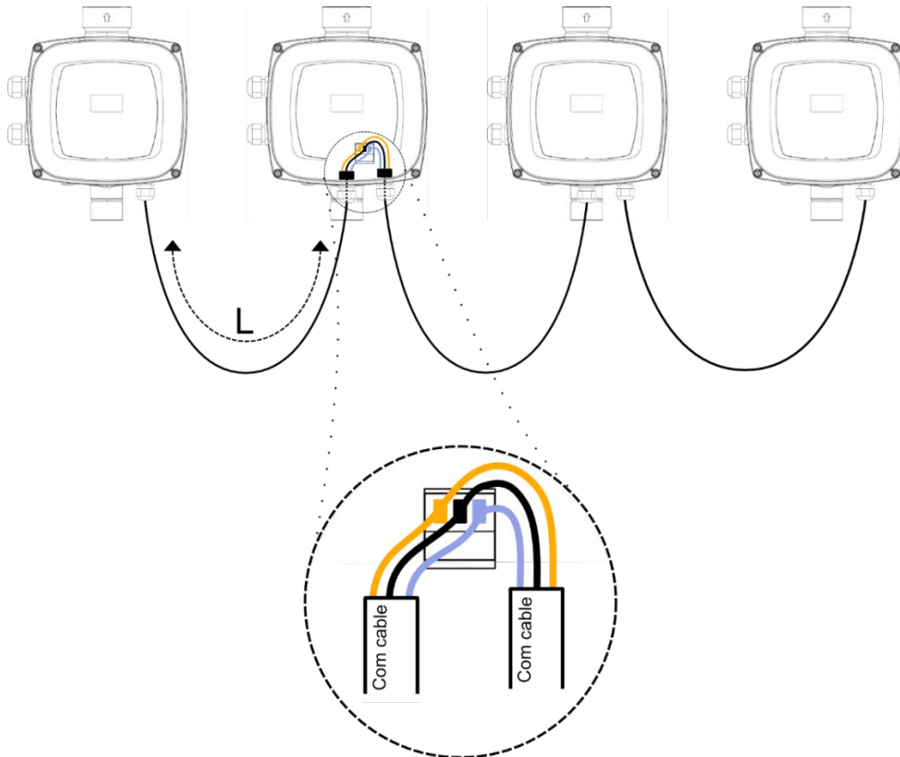
Abbildung 6: Beispiel für den Anschluss der Kommunikation Multi-Inverter mit 4 Geräten
