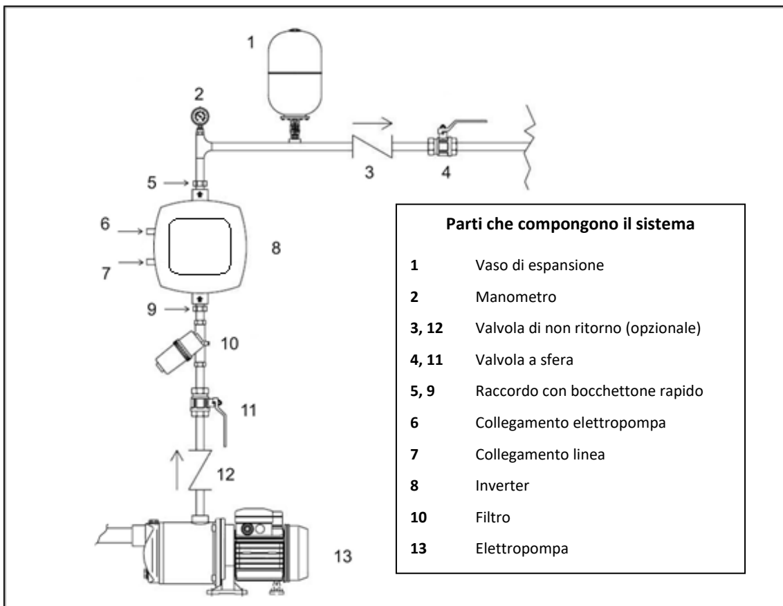
Figura 1: Installazione idraulica
