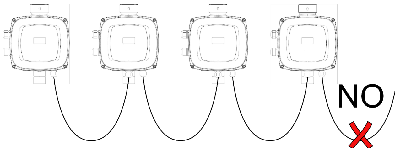
Obr. 9: Neponechávat kabel připojený pouze na jednom konci
