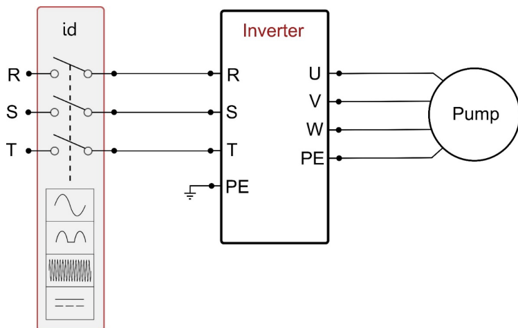
Σχήμα 3b: Παράδειγμα εγκατάστασης με τριφασική τροφοδοσία
