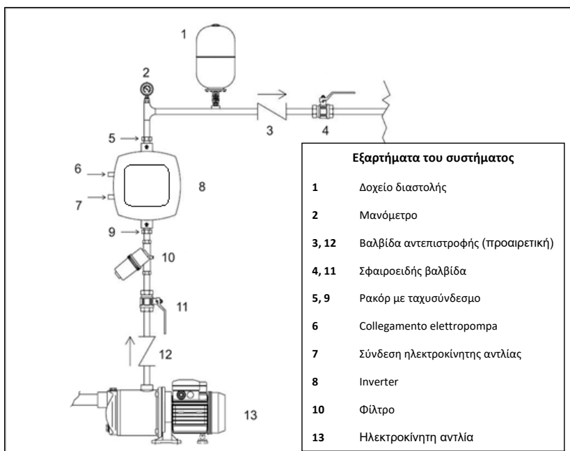
Σχήμα 1: Υδραυλική εγκατάσταση
