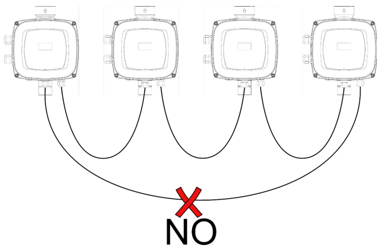
Σχήμα 7: Μην κάνετε σύνδεση δακτυλίου
