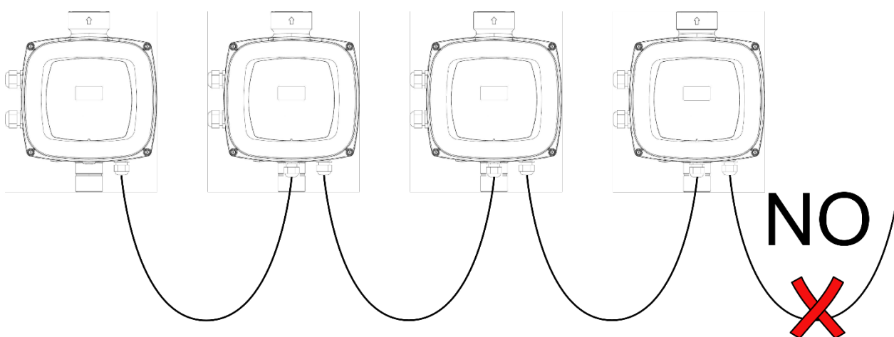
Figura 9: Não deixar cabos ligados a uma só extremidade
